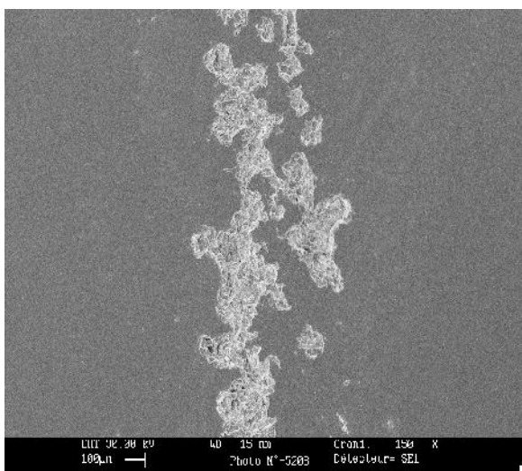
Figure II-18 : Endommagement discontinu pour une d_{tir}=30mm
