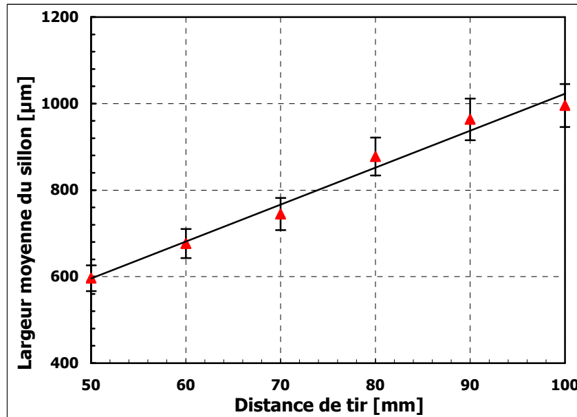
Figure II-30 : Evolution de la largeur moyenne de la saignée
