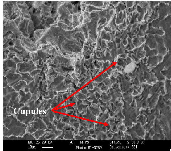
Figure II-57 : Faciès de rupture ductile et attaque en phase d'amorçage. Zoom 1
