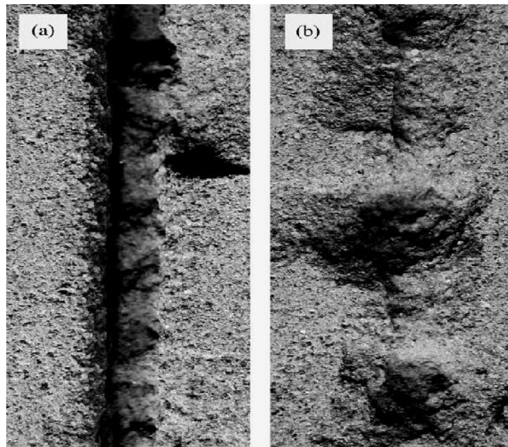
Figure II-7 : Impact sur un échantillon en grès pour : d_{tir}=60\text{mm} , d_{buse}=1.19\text{mm} , V_a=1\text{m/min} , P_c=50\text{MPa} a) dans le cas d'un jet d'eau modulé : profondeur de découpe= 3.2\text{mm} b) dans le cas d'un jet d'eau pure : profondeur de découpe= 6.8\text{mm} . [9]
