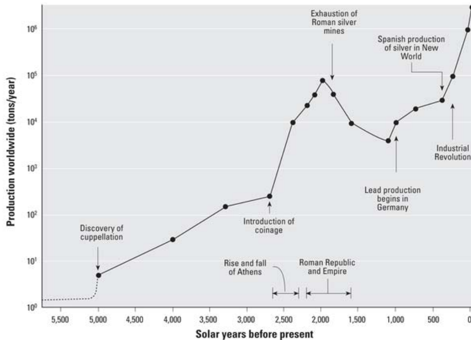
Figure 1 : Estimation de l'évolution de la production du plomb depuis 5000 ans (Settle D. and Patterson C. 1980)
