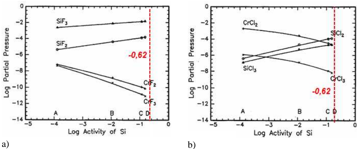
a) b) Figure V-8 : Composition de la phase gazeuse calculée à partir de divers mélanges Cr-Si activés à 1050°C a) soit par des fluorures, b) soit par des chlorures. L'alliage CrSi où \log(a_{Si}) = -0,62 est exclusivement siliciurant s'il est activé par des fluorures.
