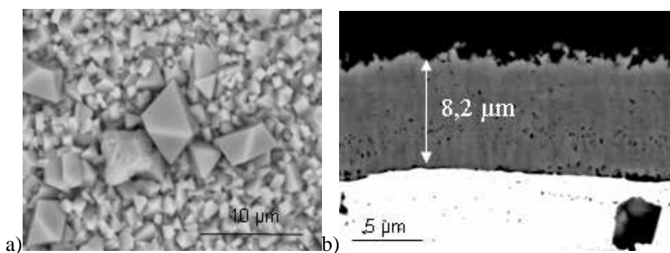
Figure IV-14 : Micrographies a) en surface après 100h d'oxydation sous Fe/FeO suivi de 100h d'oxydation sous air et b) en section après 100h d'oxydation sous FeO/Fe 3 O 4 suivi de 100h d'oxydation sous air à 1050°C.
