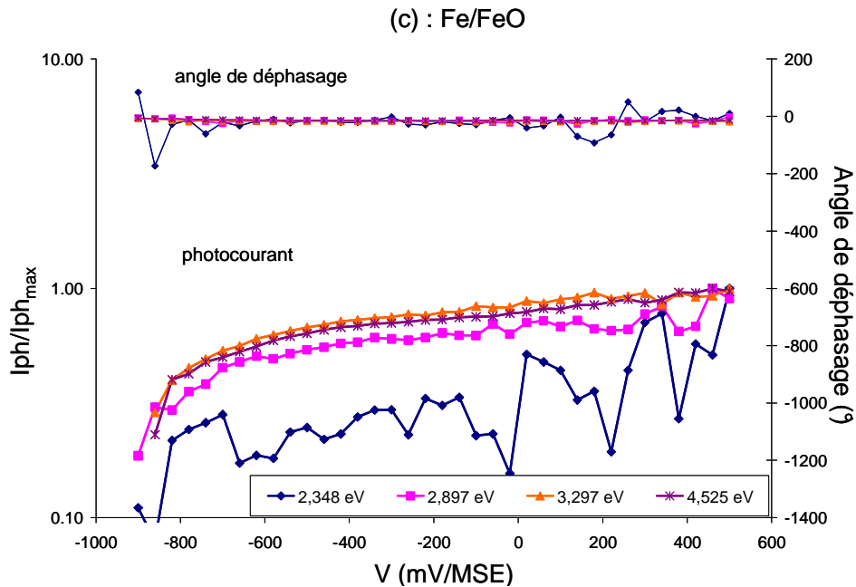
Figure IV-11 : Photocourant en fonction du potentiel à six valeurs d'énergie du rayonnement incident pour l'alliage HR120 oxydé sous faible P_{O_2} à 1050°C durant 20 minutes en présence des tampons Ni/NiO (a), FeO/Fe 3 O 4 (b) et Fe/FeO (c)
