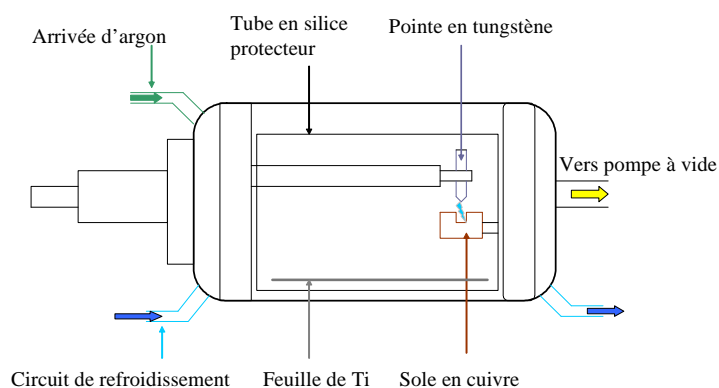
Figure II-2 : Schéma de principe du four à arc.
