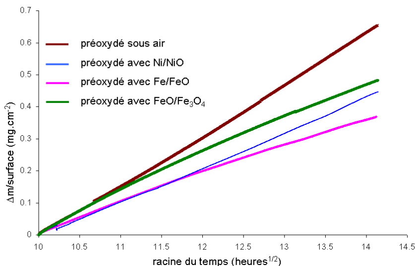
Figure IV-13 : Prise de masse en fonction de la racine carrée du temps (tracée à partir de t = 100 heures) lors de l'oxydation sous air d'échantillons de HR120 préoxydés 100 heures à 1050°C
