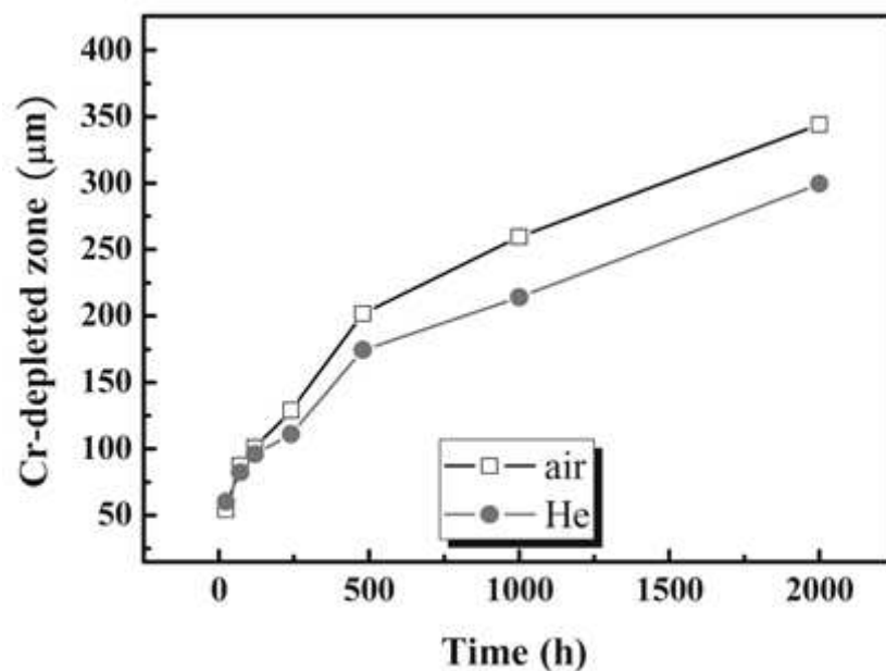
Figure I-14 : Longueur de la zone appauvrie en chrome sous air et sous He impur
