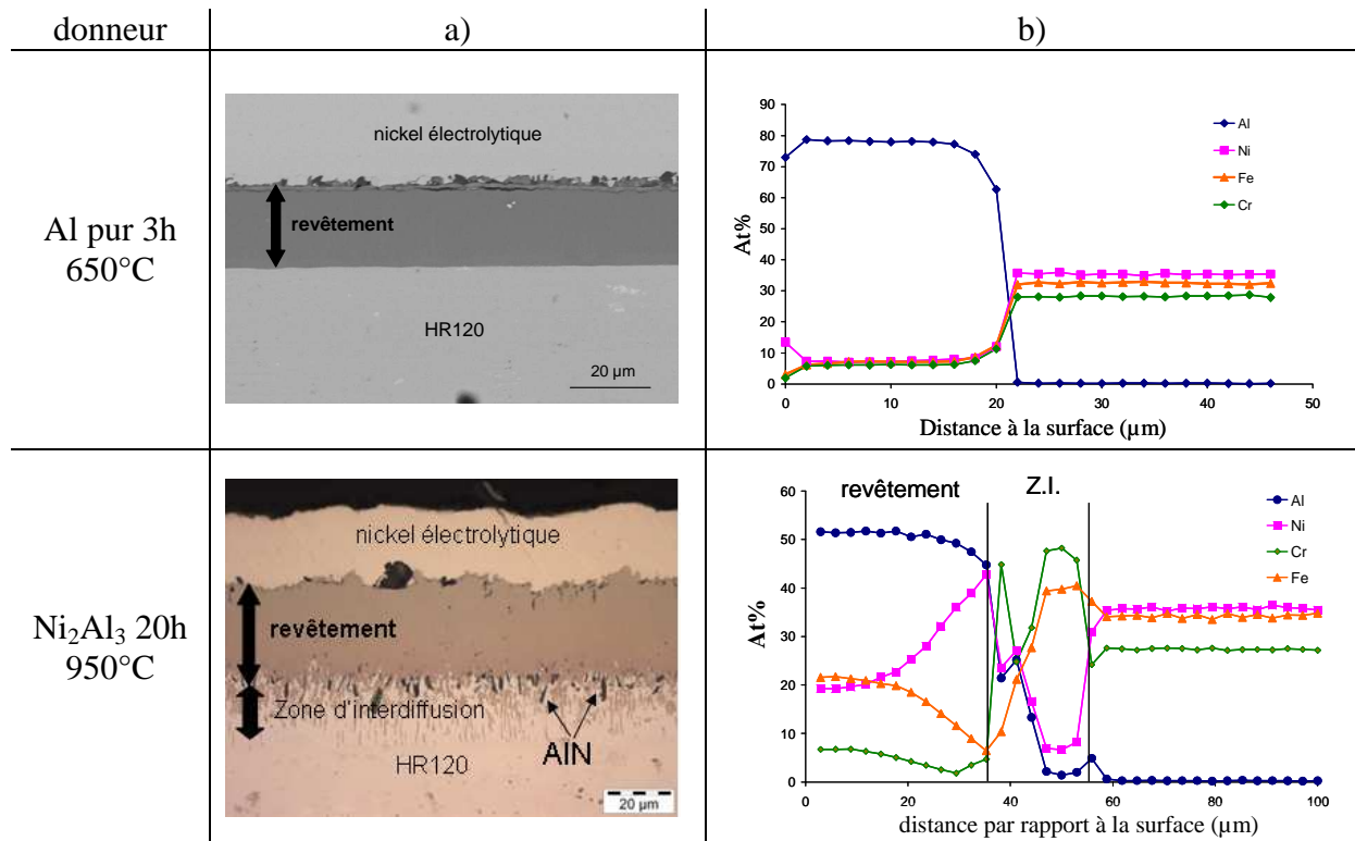
Figure V-22 : Micrographie MEB (a) et profil de concentration (b) du revêtement d'aluminisation après 3 heures de traitement à 650°C et 20h de traitement à 950°C
