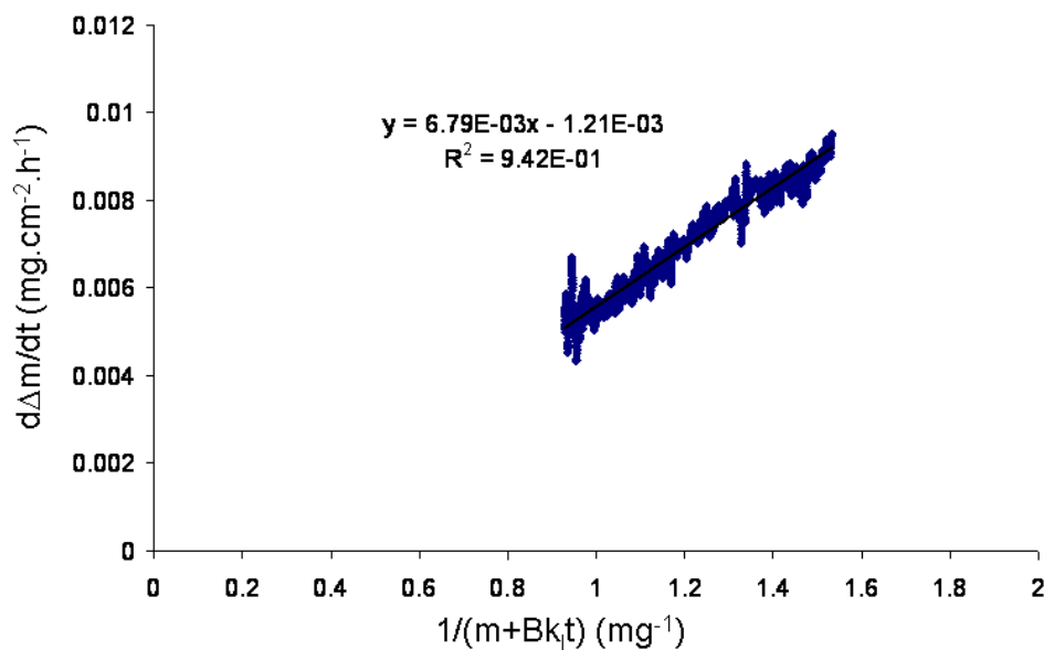
Figure III-12 : Tracé de d(\Delta m)/dt en fonction de 1/(m+k_l t) dans le cas de l'alliage HR120 oxydé 100 heures à 1050°C
