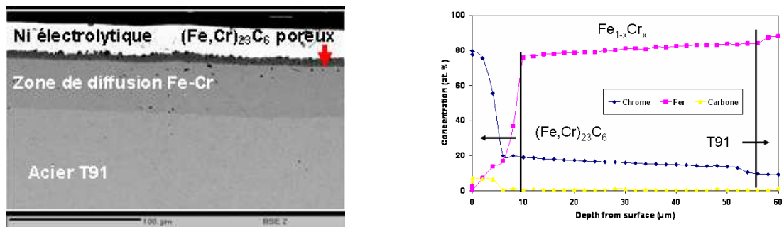
Figure I-27 : Section métallographique (MEB) et profil de diffusion (WDS) des éléments majeurs dans l'épaisseur de revêtement formé à partir du "pack" suivant : 75Fe 30 Cr 70 – 25Al 2 O 3 (wt. %) et 17 mg CrCl 3 . Le traitement a été réalisé à 980°C pendant 4 h [88]
