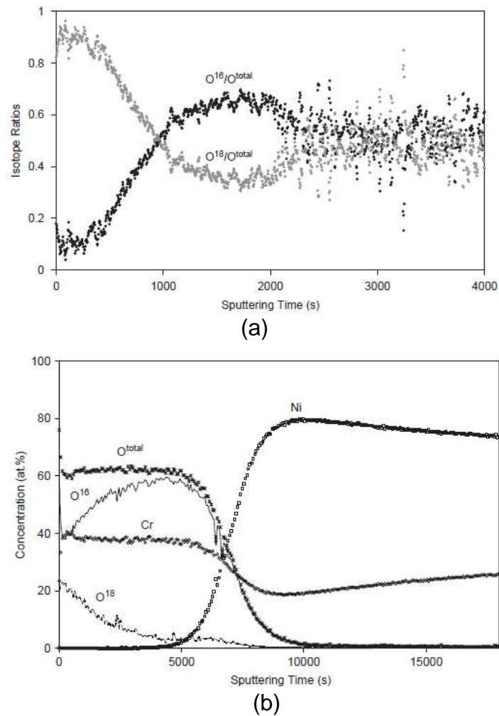
Figure I-22 : Profils isotopiques de l'oxygène mesuré par SNMS après oxydation à 1050°C de Ni-25Cr [63]. (a) première étape 30 minutes dans Ar-20% ^{16}O_2 , seconde étape 2h dans Ar – 20% ^{18}O_2 . (b) première étape 30 minutes dans Ar-20% H_2^{16}O , seconde étape 2h dans Ar – 20% H_2^{18}O
