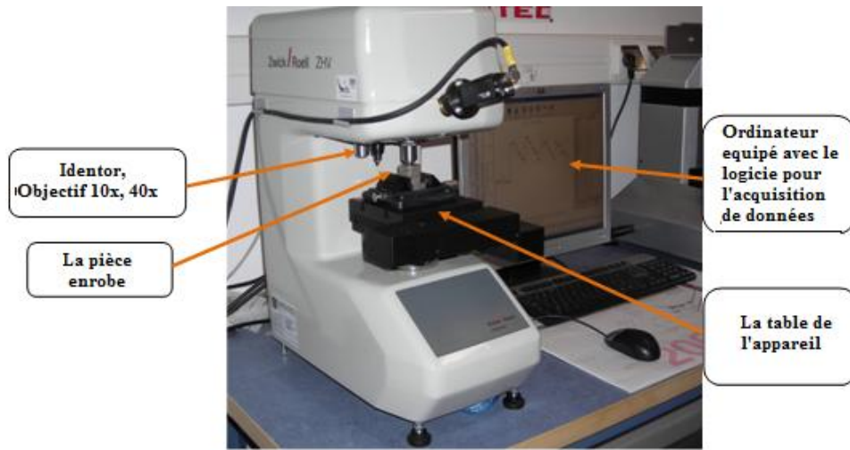
Fig. 3.21 Appareil de mesure de micro-dureté Zwick/Roell ZHV
