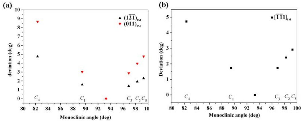
Fig. 8 Écarts angulaires de (a) plans (1\bar{2}\bar{1})_{1M} (relation de Pitsch) et (011)_{1M} (relation de K-S) et (b) direction [\bar{1}\bar{1}1]_{1M} dans les 5 sous cellules (C1, C2, ..., C5) par rapport à ceux de la cellule moyenne 1M.
