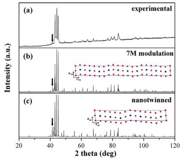
Fig.11 Diagrammes XRD pour la martensite modulée: (a) mesuré à -30^{\circ}\text{C} ; (b) recalculé avec la superstructure 7M(IC); (c) recalculé avec la cellule élémentaire tétragonale de nanomacles combinées. Les encadrés dans les figures montrent les cellules élémentaires des deux structures.
