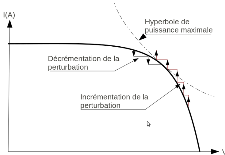
FIGURE 4.25 – Représentation du trajet effectué par un « Perturb and Observe » sur la caractéristique du panneau. Lorsque le maximum local est dépassé, il y a inversion de la perturbation et le système se stabilise autour du MPP.
