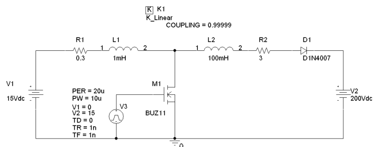
FIGURE 5.14 – Schéma de simulation du Boost à couplage magnétique.
