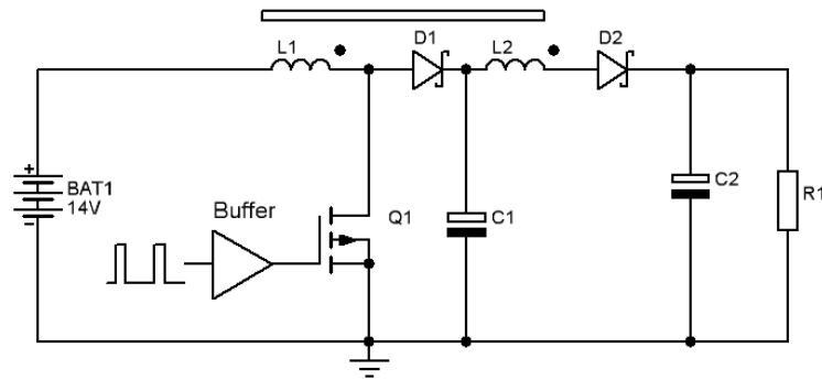
FIGURE 4.11 – Schéma d'un boost à récupération basé sur un Boost classique associé à un circuit secondaire élévateur.
