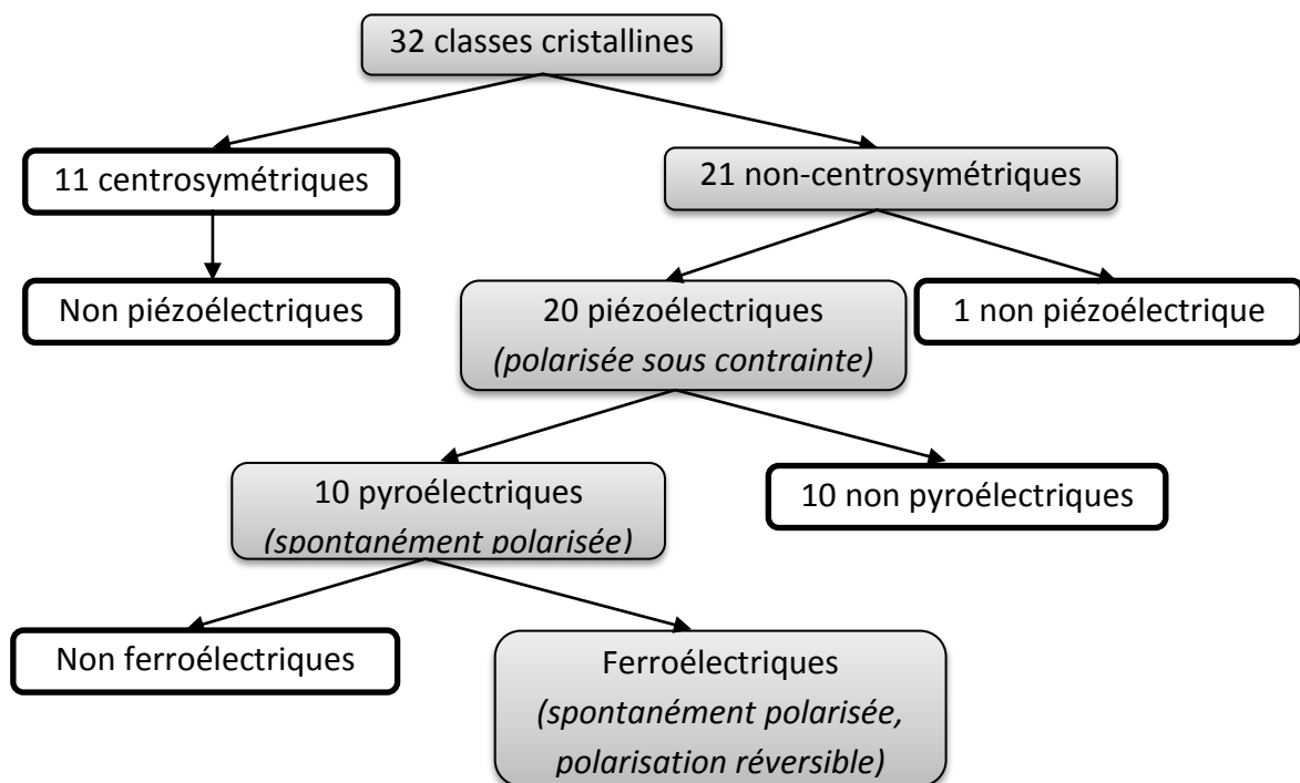
Figure 2.1-1 : Classification des systèmes cristallins.
