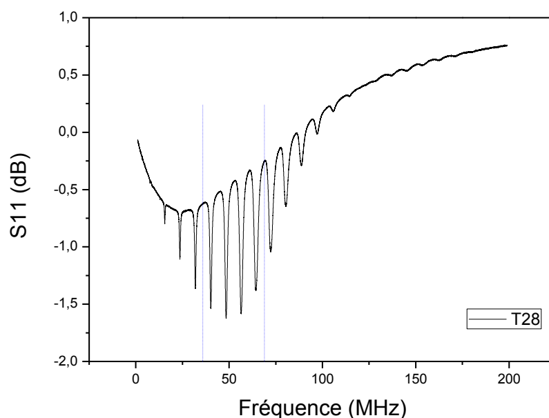
Figure 3.5-3: Spectre S11 de l'OMR imprimé 6000 \mu\text{m} sur un film de P(VDF-TrFE) de 6.3 \mu\text{m} d'épaisseur sur PET.
