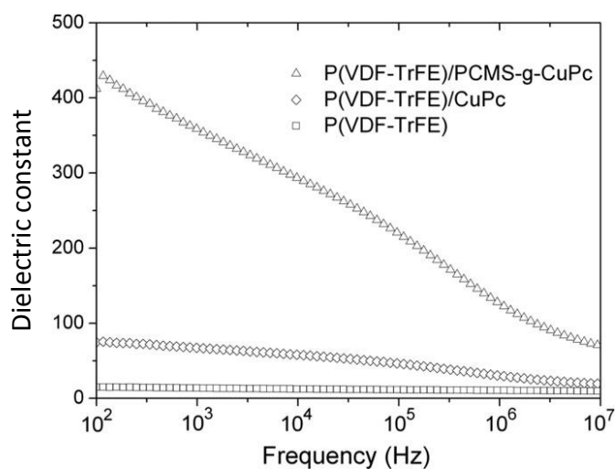
Figure 2.1-23 : Constante diélectrique à température ambiante en fonction de la fréquence pour les films par « solution casting » de P(VDF-TrFE)/PCMS-g-CuPc, P(VDF-TrFE)/CuPc, et P(VDF-TrFE) pur, extraite de [80].
