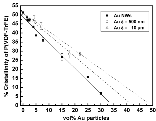
Figure 2.1-19: Taux de cristallinité de la matrice de P(VDF-TrFE) en fonction de la fraction volumique d'Au avec la taille de particule: (■) NFs de 200 nm de diamètre et 45 \mu\text{m} de largeur, (○) particules de 500 nm de diamètre, ( \Delta ) particules de 10 \mu\text{m} de diamètre, figure extraite de [70].
