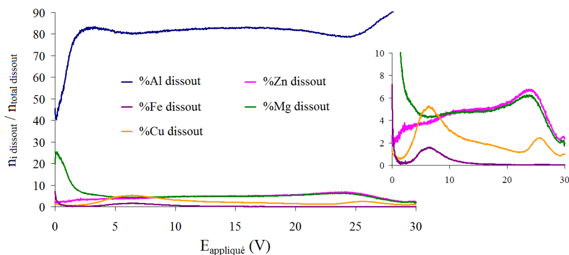
Figure 136 : Evolution du pourcentage dissous d'un élément i par rapport à la quantité totale dissoute en fonction du potentiel appliqué à l'alliage 7050 dans H_2SO_4 200 g/l
