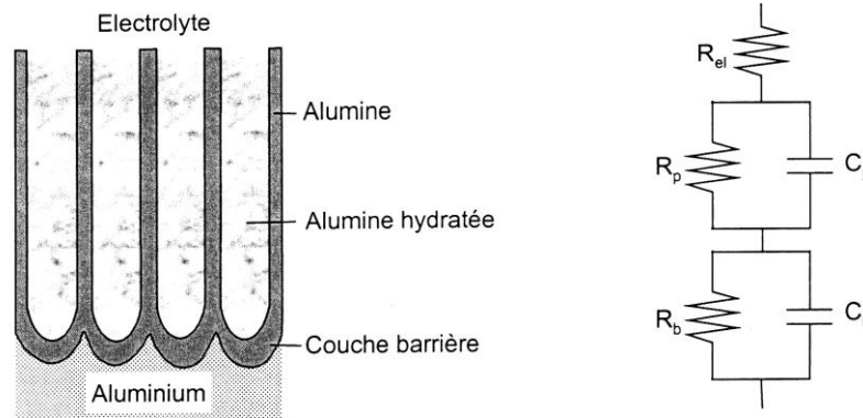
Figure 28 : Circuit électrique équivalent d'une couche anodique colmatée d'après Hitzig et ses collaborateurs [9]
