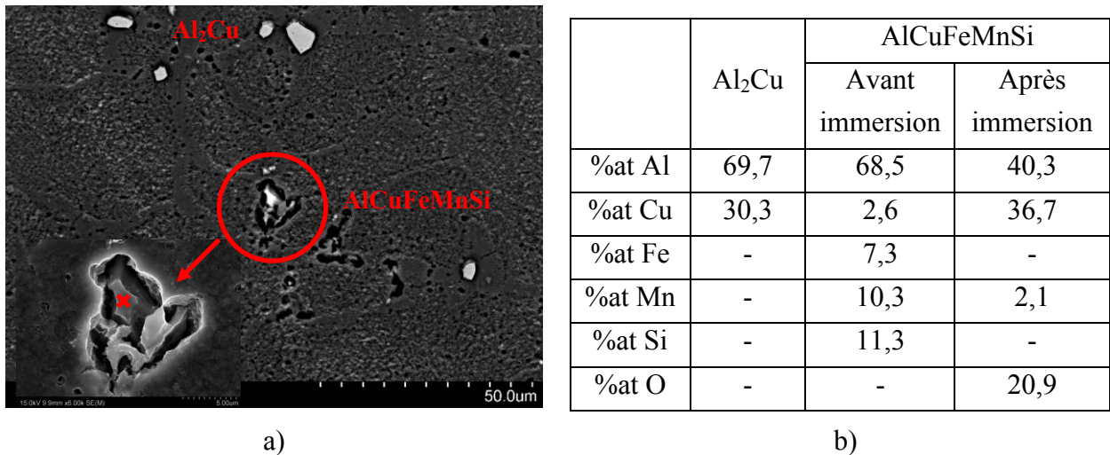
Figure 144 : Micrographies de l'alliage 2214 (a) et composition EDS (b) des phases intermétalliques après 15 minutes d'immersion dans la solution Isoprep 161
