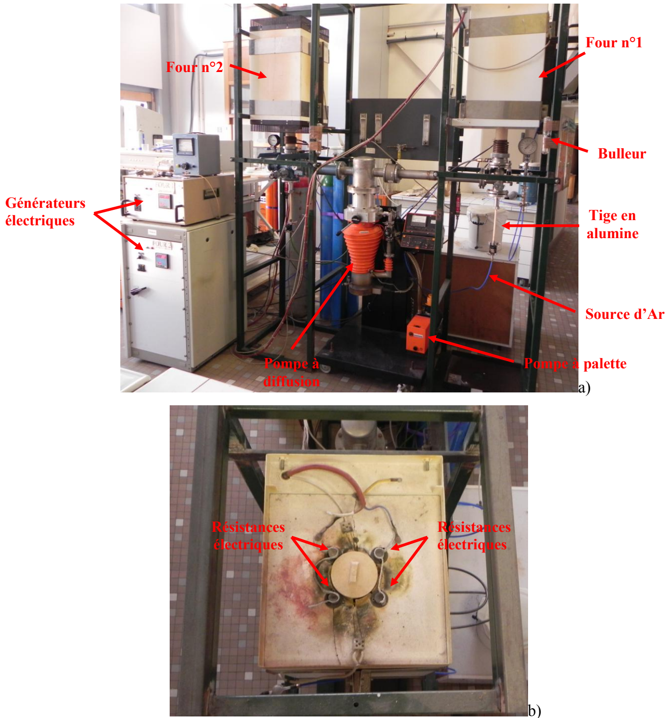
Figure 24 : Fours verticaux pyrox : vue de face (a), vue de dessus (b)
