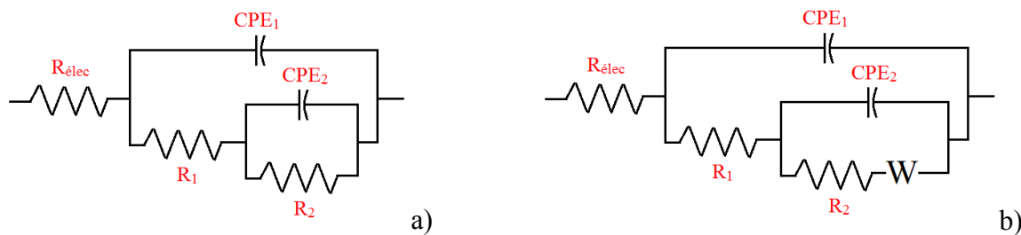
Figure 96 : Circuits électriques équivalents utilisés pour modéliser les résultats à t < 18 heures d'immersion (a) et t > 18 heures d'immersion (b)
