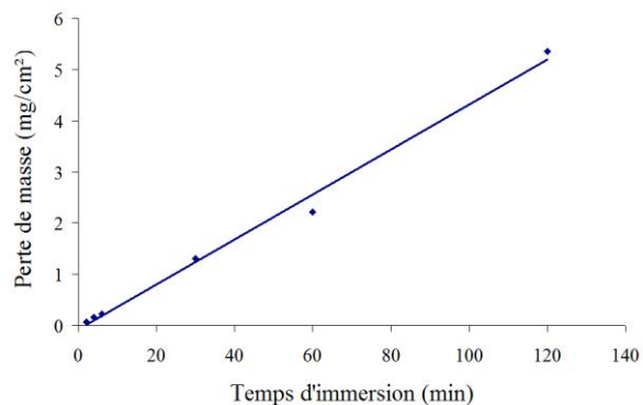
Figure 163 : Evolution de la perte de masse de l'alliage 7050 en fonction du temps d'immersion dans la solution commerciale de décapage Ardrox 295GD
