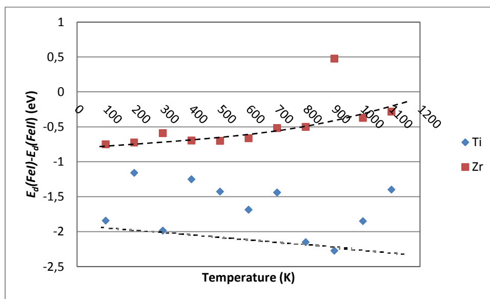
Fig.7 Les différences des énergies (en eV) entre les substitutions dans des sites FeI et FeII
