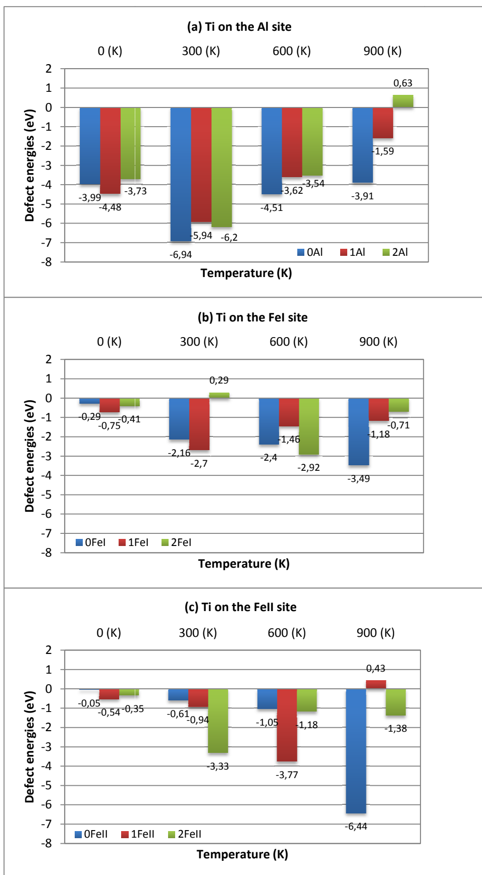
Fig.8 Energies de défauts pour le Ti pour différentes température 300, 600, 900K sur différents sites (a) Al (b) FeI et (c) FeII en tenant compte des distances suivant l'interface.
