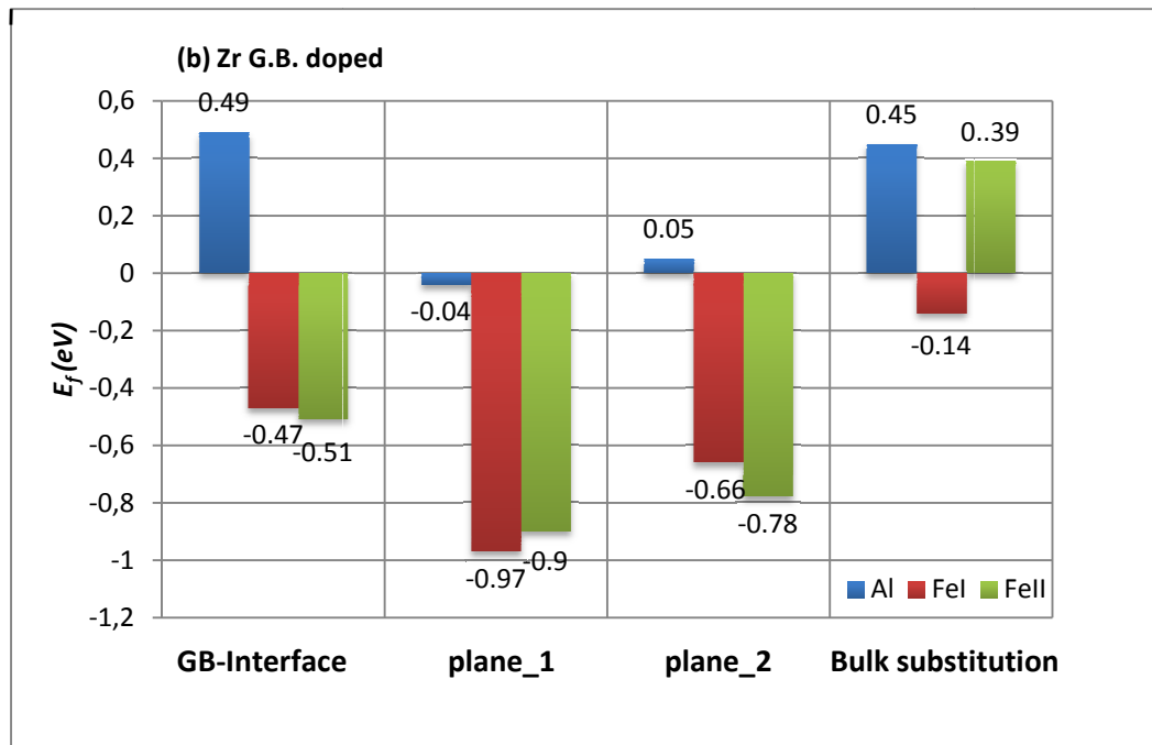
Fig. 5. Énergies de formation des impuretés (en eV) pour différents sites de substitution dans (a) le système dopé avec du titane (b) système dopé avec du zirconium.
