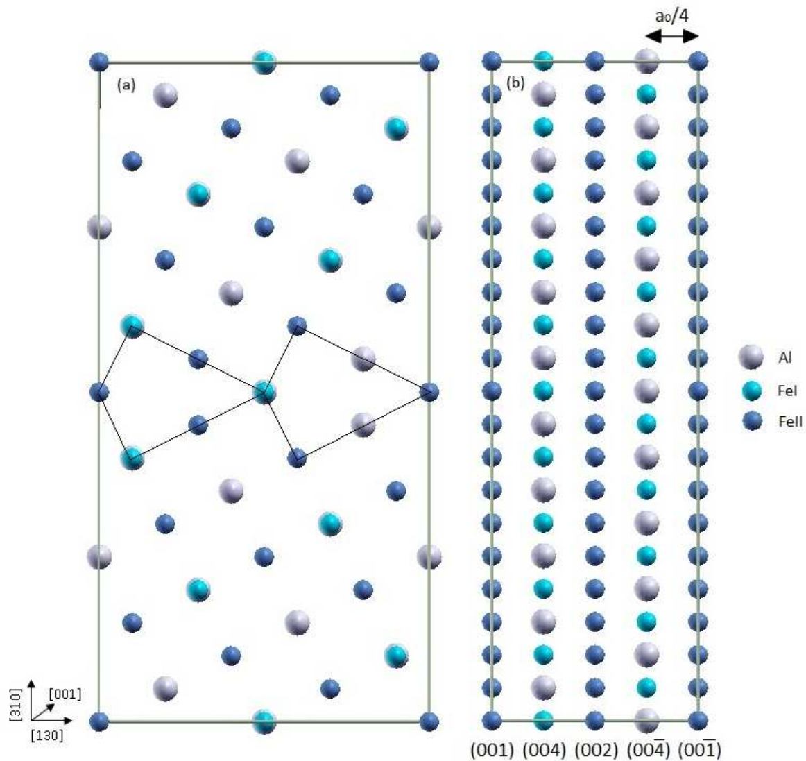
Fig. 3 La structure atomique du joint de grains \Sigma 5 (310) [001] dans l'intermétallique D0_3 - Fe_3Al (a) vue le long de la direction [001] (b) vue le long de la direction [130] .
