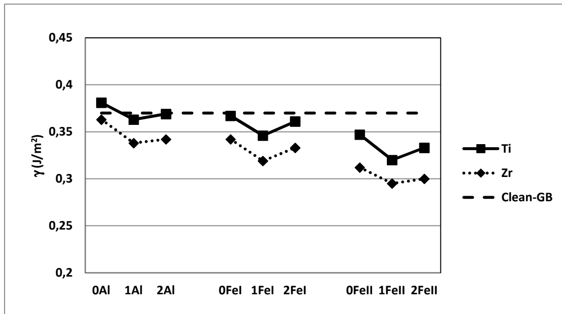
Fig. 6. Les énergies d'interface (en J/m 2 ) calculées pour les joint de grains dopé et non-dopé.
