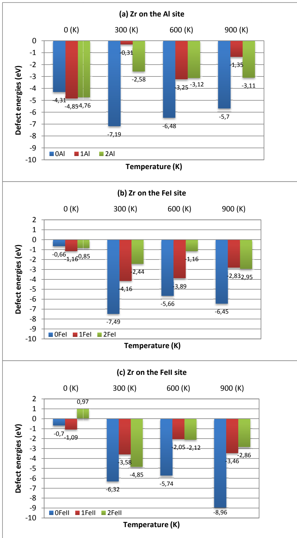
Fig. 9 Energies de défauts pour le Zr pour différentes température 300, 600, 900K sur différents sites (a) Al (b) FeI et (c) FeII en tenant compte des distances suivant l'interface.
