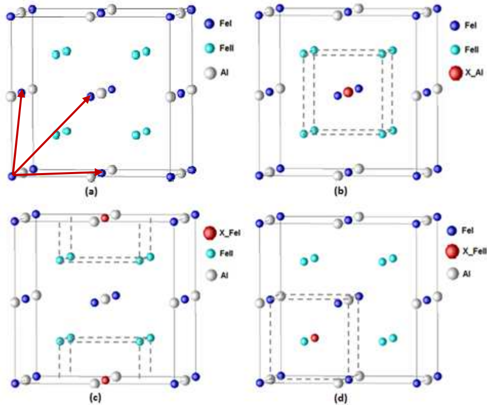
Fig. 1. (a) La structure D0_3\text{-Fe}_3\text{Al} non-dopée et les trois défauts de substitutions ainsi que les lacune sur les sites (b) Al (c) FeI et (d) FeII.
