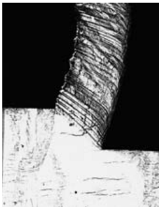
Copeau continu
