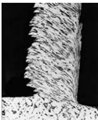
Copeau segmenté
