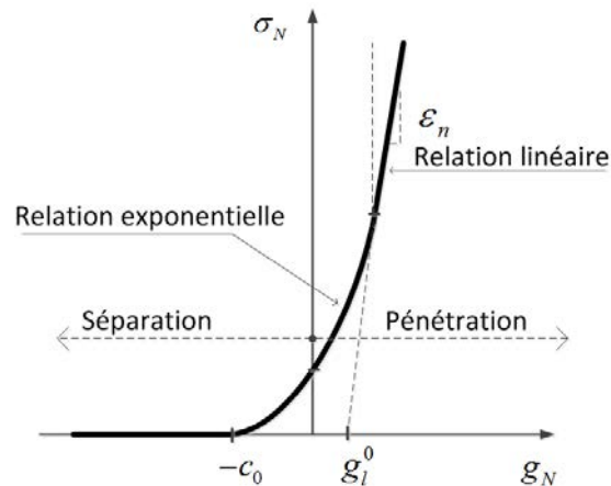
Figure 4. 7 : Relation entre la pression de contact et la distance minimale de contact normal.
