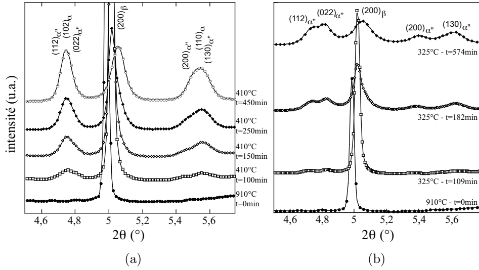
FIG. 2.20: Evolution des diffractogrammes au cours des maintiens à (a) 410°C et (b) 325°C. Le pic (200)_{\beta} est tronqué sur la figure (a)
