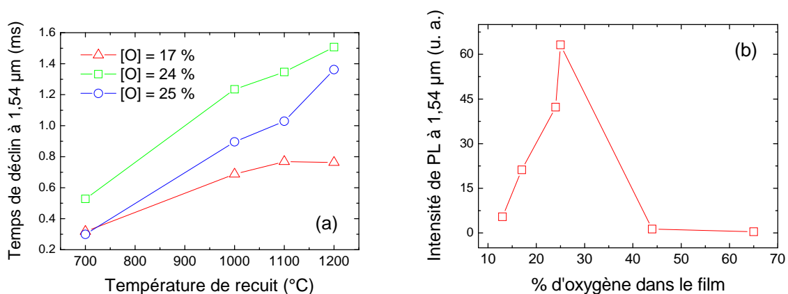
Figure 3-25 : (a) Evolution du temps de déclin de l'erbium à 1,54 \mu\text{m} mesuré à 300 \text{ K} en fonction de la température de recuit pour des films de \text{SiO}_x\text{N}_y:\text{Er} contenant entre 17 % et 25 % d'oxygène. L'excitation des ions \text{Er}^{3+} est indirecte et se fait à 355 \text{ nm} . (b) Evolution de l'intensité de PL de l'erbium à 1,54 \mu\text{m} mesurée à 300 \text{ K} pour une excitation à 325 \text{ nm} en fonction du pourcentage d'oxygène contenu dans des films de \text{SiO}_x\text{N}_y:\text{Er} recuits à 1200 \text{ }^\circ\text{C} .
