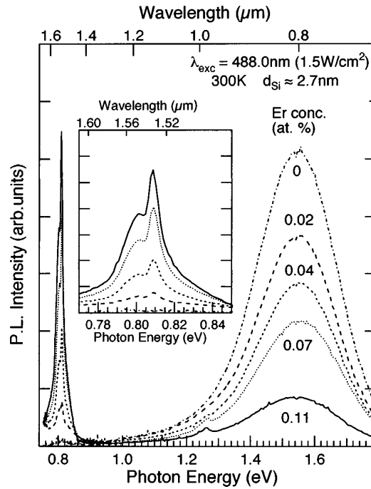
Figure 1-5 : Evolution des spectres de PL d'échantillons de silice contenant des nanocristaux de silicium et des ions \text{Er}^{3+} en fonction de la concentration en erbium. D'après [45].
