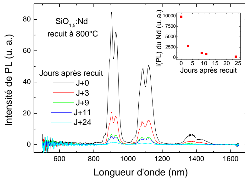
Figure 5-10 : Spectre de PL continue réalisé à température ambiante avec une excitation à 325 nm sur le film de \text{SiO}_{1.5}:\text{Nd} recuit à 800^\circ\text{C} (dopage à 4 at.%) en fonction du nombre de jours écoulés depuis le traitement thermique de l'échantillon. En encart : Intensité de PL du Nd intégrée entre 800 et 1550 nm en fonction du nombre de jours écoulés depuis le recuit.
