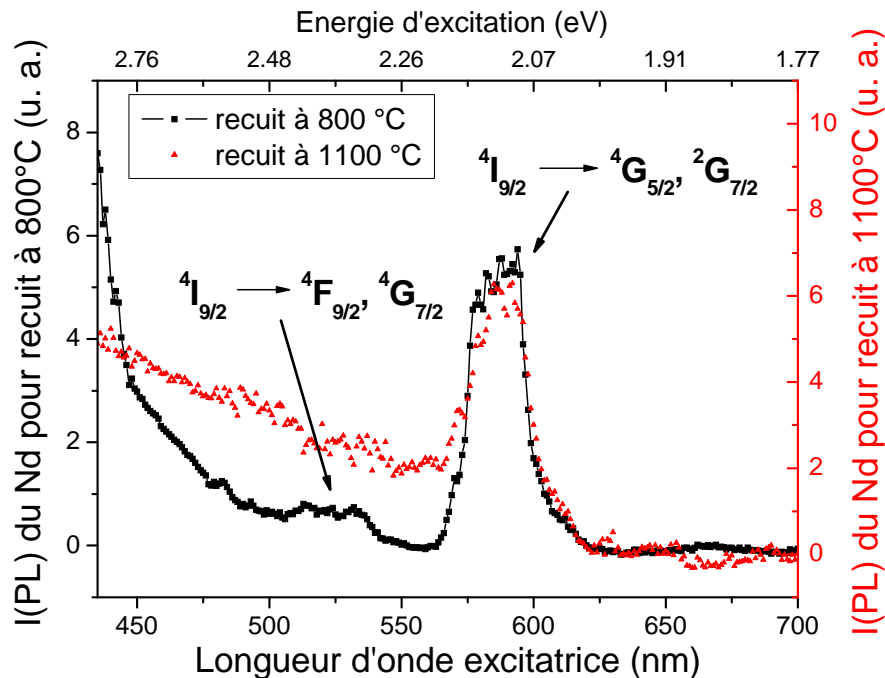
Figure 5-13 : Spectres de PLE du Nd mesurés à 920\text{ nm} à 300\text{ K} sur les films de \text{SiO}_{1.5}:\text{Nd} dopés à 4\text{ at.}\% et recuits à 800 et 1100\text{ }^\circ\text{C} . La puissance moyenne du laser vaut 50\text{ mW} .
