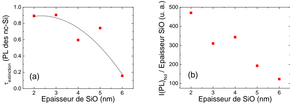
Figure 5-4 : (a) Coefficient d'extinction de la PL des nc-Si défini par la relation (5-1) en fonction de l'épaisseur de la couche de SiO dans les multicouches SiO/SiO 2 recuites à 1100 °C. La ligne continue est un guide pour l'œil. (b) Rapport de l'intensité de PL des ions \text{Nd}^{3+} par l'épaisseur de SiO en fonction de l'épaisseur de la couche de SiO des multicouches SiO/SiO 2 dopées au Nd et recuites à 1100 °C. La longueur d'onde d'excitation vaut 325 nm et l'intensité de PL du Nd est obtenue par intégration du signal à 300 K entre 850 et 1000 nm (transition {}^4\text{F}_{3/2} \rightarrow {}^4\text{I}_{9/2} ) après soustraction de la contribution des nc-Si.
