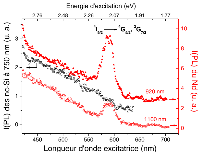
Figure 4-14 : Spectres d'excitation de PL du Nd (à 920 et 1100 nm) et des nc-Si (à 750 nm) mesurés à température ambiante sur un film de SiO 1,5 :Nd (dopage 4 at.%) recuit à 1100 °C. La puissance moyenne du laser est égale à 50 mW.
