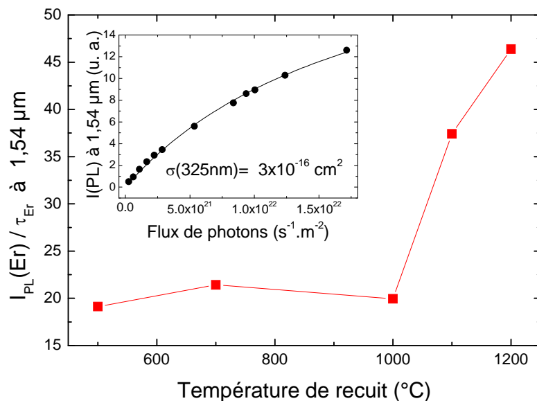
Figure 3-28 : Evolution du rapport I_{\text{PL}} / \tau_{\text{Er}} calculé pour des mesures réalisées à 1,54 μm à température ambiante en fonction de la température de recuit pour le film de \text{SiO}_x\text{N}_y:\text{Er} contenant 25 % d'oxygène. En encart : Evolution de l'intensité de PL de l'erbium à 1,54 μm en fonction du flux de photons excitateurs pour le film de \text{SiO}_x\text{N}_y:\text{Er} recuit à 1200 °C et contenant 25 % d'oxygène. Les mesures sont réalisées à 300 K avec une excitation à 325 nm.
