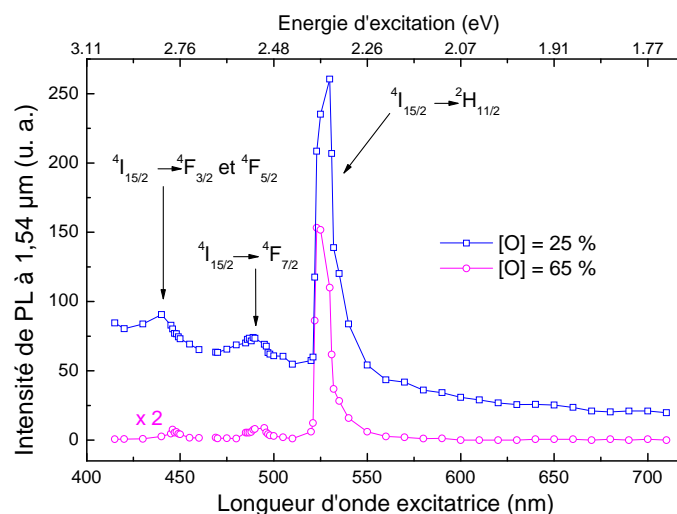
Figure 3-26 : Spectres d'excitation de photoluminescence mesurés à température ambiante et à 1,54 \mu\text{m} des films de \text{SiO}_x\text{N}_y:\text{Er} recuit à 1200^\circ\text{C} et contenant 25 % et 65 % d'oxygène.
