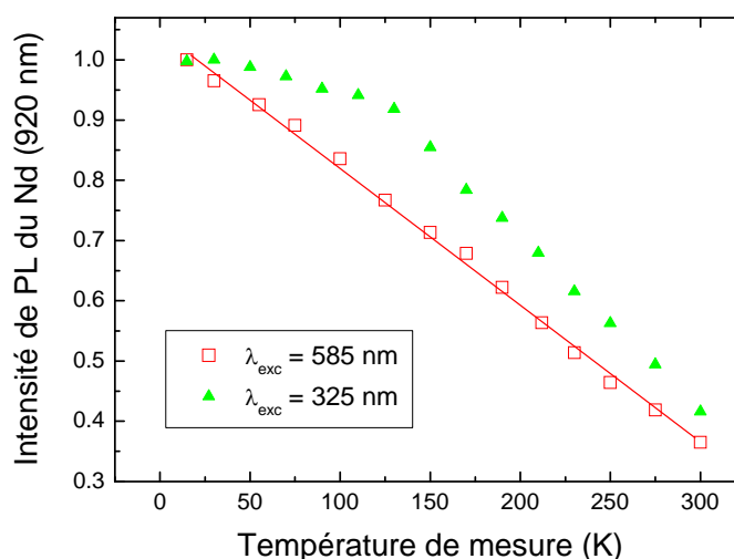
Figure 6-14 : Intensité de PL des ions \text{Nd}^{3+} à 920 nm obtenues après excitations directe (à 585 nm) et indirecte (à 325 nm) en fonction de la température de mesure pour le film de \text{SiO}_{1.5}:\text{Nd} contenant des nc-Si et dopé à 1 at.% en Nd.
