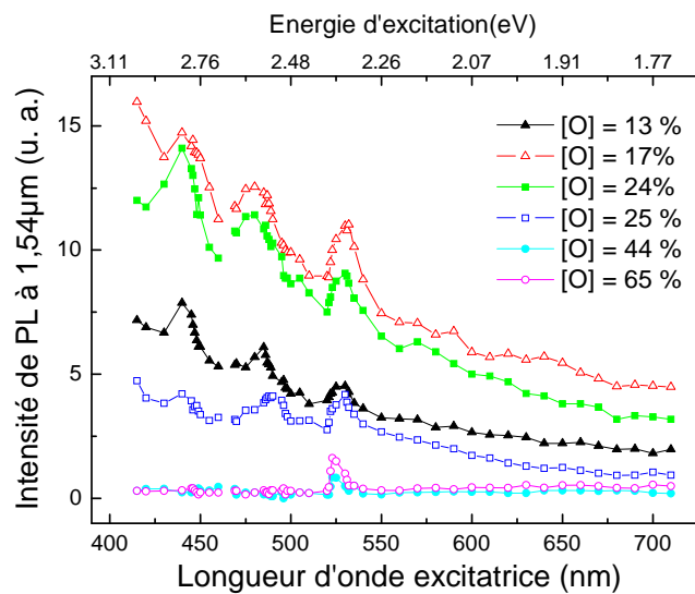
Figure 3-32 : Spectres de PLE des films contenant entre 13 % et 65 % d'oxygène recuits à 700 °C (a). Le signal est mesuré à 1,54 µm et la température de mesure est de 300 K.
