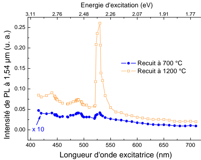
Figure 3-31 : Spectres d'excitation de photoluminescence réalisés à température ambiante à 1,54 µm sur les films de \text{SiO}_x\text{N}_y:\text{Er} contenant 25 % d'oxygène et recuits à 700 °C et 1200 °C.
