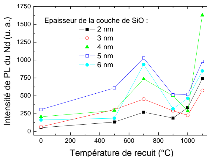
Figure 5-17 : Intensité de PL du Nd intégrée entre 1000 et 1250 nm (transition {}^4\text{F}_{3/2} \rightarrow {}^4\text{I}_{11/2} ) en fonction de la température de recuit pour les multicouches \text{SiO}/\text{SiO}_2 dopées au Nd (0,5 at.%) dont l'épaisseur de \text{SiO} varie de 2 à 6 nm. Les mesures sont effectuées à température ambiante avec une excitation à 325 nm non résonante avec les états électroniques du Nd.
