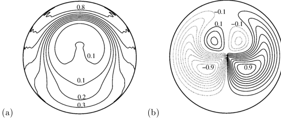
FIGURE 5.4: Iso-contours du taux de cisaillement pour un fluide Newtonien à Re = 2000 et \varepsilon_0 = 10^{-3} : (a) Contours de \left| \partial \tilde{W}_b / \partial r \right| / \left| \partial \tilde{W}_b / \partial r \right|_{max} , avec \left| \partial \tilde{W}_b / \partial r \right|_{max} = 4.05 . (b) Contours de \left[ (1/r) \partial \tilde{W}_b / \partial \theta \right] / \left[ (1/r) \partial \tilde{W}_b / \partial \theta \right]_{max} , avec \left[ (1/r) \partial \tilde{W}_b / \partial \theta \right]_{max} = 0.737 .
