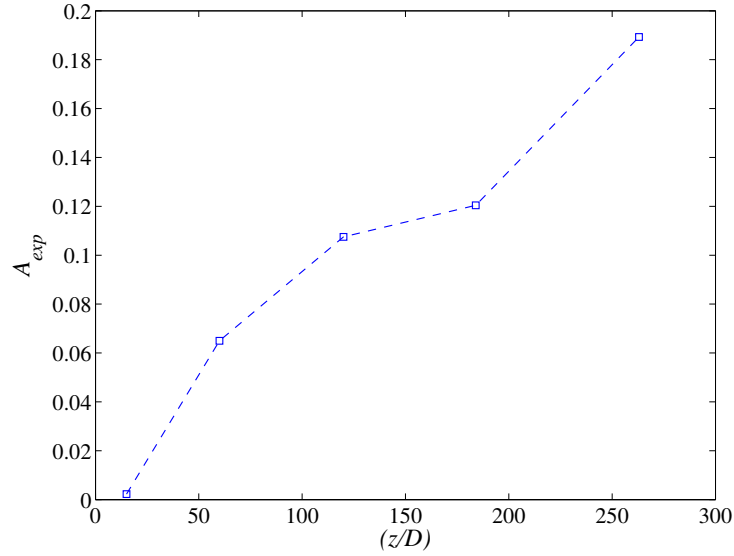
FIGURE 1.7: Variation de l'asymétrie en fonction de la coordonnée axiale de la conduite z/D pour une solution de Carbopol modélisée par une loi de Carreau-Yasuda avec \hat{\lambda} = 0.8 et n_c = 0.6 pour un Reynolds de paroi Re_w = 3400 .
