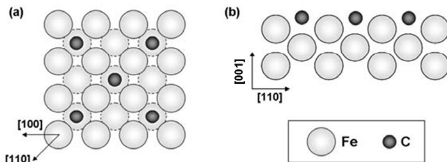
Figure II-3 – Modèle structural de la reconstruction c(2 \times 2) après ségrégation du C à la surface du Fe(001) ; (a) vue de dessus, (b) vue en coupe. D'après [16].
