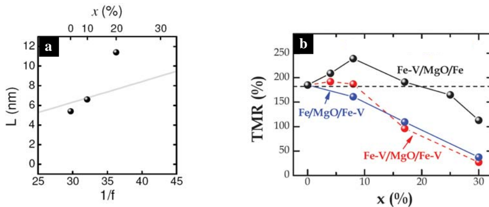
Figure I-12 – (a) Distance moyenne L entre dislocations à l'interface inférieure \text{Fe-V}/\text{MgO} (points noirs) mesurée dans des JTM's \text{Fe}_{1-x}\text{V}_x/\text{MgO}/\text{Fe}(001) , tracée en fonction du désaccord paramétrique f et de la concentration x de vanadium. D'après [2]; (b) Variation de la TMR à température ambiante avec la concentration x de vanadium dans différentes séries de JTM's. D'après [38].
