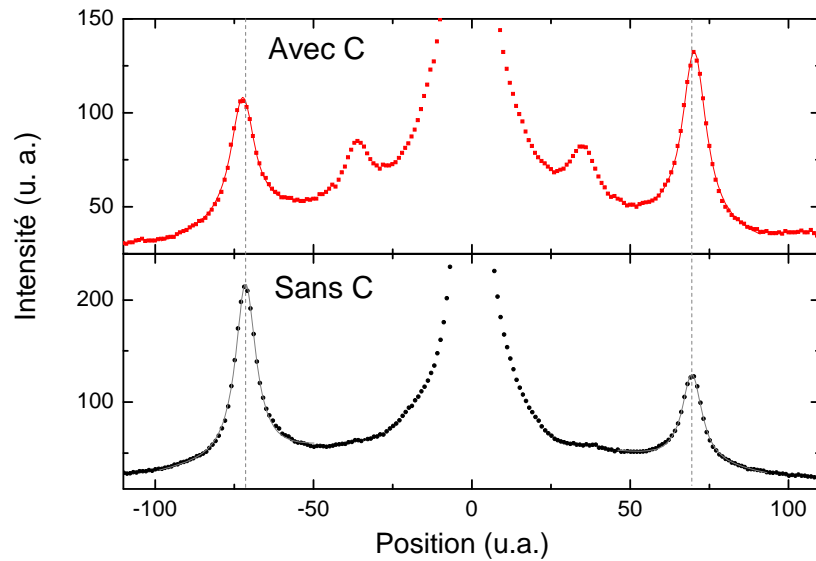
Figure II-2 – Profils d'intensité RHEED perpendiculairement aux raies de diffraction, dans l'azimut [11] d'une surface de Fe(001) propre (en bas) ou présentant une reconstruction c(2 \times 2) due à la présence de carbone (en haut). Les points correspondent aux valeurs d'intensité mesurées, et les lignes à un ajustement par des courbes lorentziennes avec un fond linéaire.
