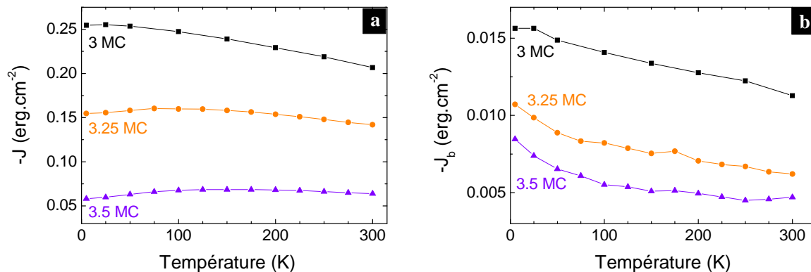
Figure IV-24 – Evolution en température des constantes de couplage (a) bilinéaire J et (b) biquadratique J_b dans des échantillons Fe(50 nm)/MgO( t_{MgO} )/Fe(5 nm).
