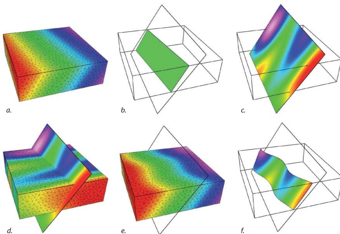
FIGURE 1.19 – Méthode de perturbation 2D d’une surface implicite. Champ scalaire initial \mathcal{F}(x, y, z) (a.) et surface correspondante (b.). c. Le champ de perturbation \mathcal{R}(x, y, z) est généré sur une grille 2D parallèle au plan de faille. d. La perturbation est transférée à l’ensemble du domaine par projection. e. Le champ \mathcal{R}(x, y, z) est ajouté au champ de la faille \mathcal{F}(x, y, z) . f. Nouvelle géométrie de la faille.
