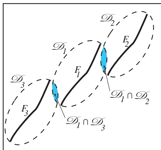
FIGURE 1.26 – Nucléation de failles secondaires dans une zone en relai. Vue de dessus de trois failles principales. L'intersection des domaines d'extension de deux failles représente une zone à forte probabilité de failles secondaires.
