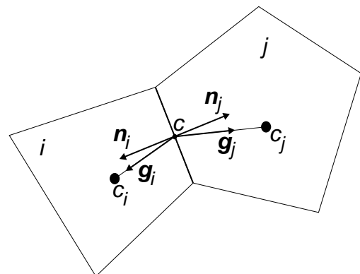
FIGURE 3.6 – Calcul de la transmissibilité entre deux primitives géométriques.
