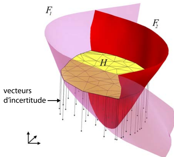
FIGURE 3 – Incertitude de type 1 induisant une incertitude de type 3. Dans le cas initial, l'horizon H se situe entre les failles F_1 et F_2 . Une simple translation de H le long de vecteurs d'incertitude peut complètement changer la configuration : H pourrait être en contact avec seulement F_1 ou F_2 et ne plus se situer entre les deux failles. D'après Cherpeau et al. [2010a].
