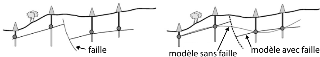
FIGURE 2 – Types d'incertitudes en modélisation structurale. a. L'incertitude de type 1 est due aux imprécisions et erreurs de mesure. La position de l'horizon est ici incertaine, sa position n'est connue que dans un intervalle. (b.) L'incertitude de type 2 est due à la variabilité naturelle intrinsèque des objets géologiques. c. L'incertitude de type 3 concerne l'existence des objets et leurs relations. Modifié d'après Wellmann et al. [2010].
