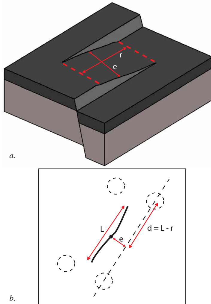
FIGURE 1.25 – Paramètres et probabilité de nucléation de failles en relié. a. Deux failles en relié peuvent être décrites par rapport à leur éloignement et leur recouvrement (schéma modifié d’après Peacock and Parfitt [2002]). b. Ces deux paramètres pourraient servir à définir des zones à forte probabilité lors de la nucléation d’une nouvelle faille (vue de dessus).
