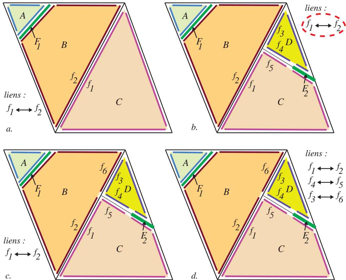
FIGURE 3.5 – Intersection partielle et mise à jour des liens (vue de dessus). a. Le tétraèdre de gauche contient trois primitives : A , B et la primitive correspondant à la faille F_1 . L'autre tétraèdre ne contient que C . b. Une faille F_2 recoupe la primitive C . La primitive D est créée. La faille F_2 ne recoupe pas complètement le tétraèdre, les faces f_4 et f_5 sont voisines. Le lien entre f_1 et f_2 existe toujours mais f_2 doit être intersectée par F_2 pour garder une cohérence entre faces. c. La face f_2 est coupée en deux, f_6 est créée. d. Les faces voisines nouvellement créées sont connectées, les faces f_3 , f_6 et f_4 , f_5 sont liés.
