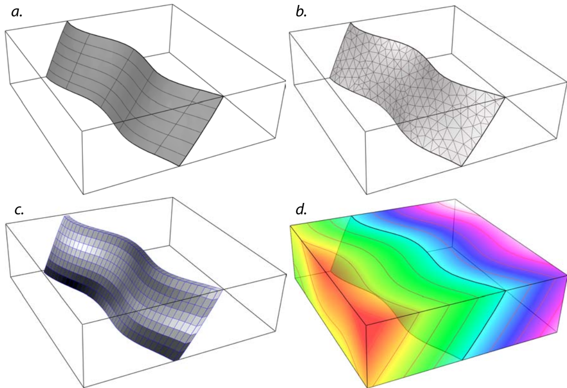
FIGURE 1.2 – Représentations d'une faille en géomodélisation. a. Objet faille proposé par Lecour et al. [2001]. Les lignes horizontales sont des génératrices, les lignes verticales constituent la "colonne vertébrale". b. Représentation par surface triangulée utilisée en modélisation explicite. c. Représentation volumique dans une grille hexaédrique, ce qui permet d'estimer les propriétés hydrauliques de la faille. d. Représentation par surface implicite (voir section 1.2 pour plus de détail).
