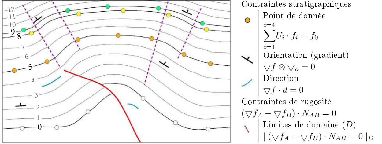
FIGURE 1.4 – Données utilisées et contraintes DSI associées pour le calcul d'un champ scalaire f . Des points de données, associées à une valeur f_0 (correspondant à un âge relatif d'une pile stratigraphique par exemple), contraignent les valeurs du champ scalaire. Des données d'orientation et de direction peuvent également être prises en compte. Enfin, des contraintes de rugosité, sur l'ensemble du modèle ou par domaine, sont ajoutées (A et B sont deux tétraèdres voisins). D'après Durand-Riard [2010].
