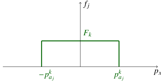
FIGURE 4.2.: Représentation de la fonction de distribution longitudinale f_j(p_x) de type water-bag simple, pour un bag k d'amplitude F_k , dans un cas symétrique, à l'équilibre.
