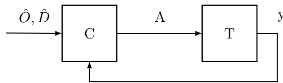
FIGURE A.9 – Schéma de la boucle de rétro-action formée avec les entrées et les sorties de l'architecture et le système cible.
