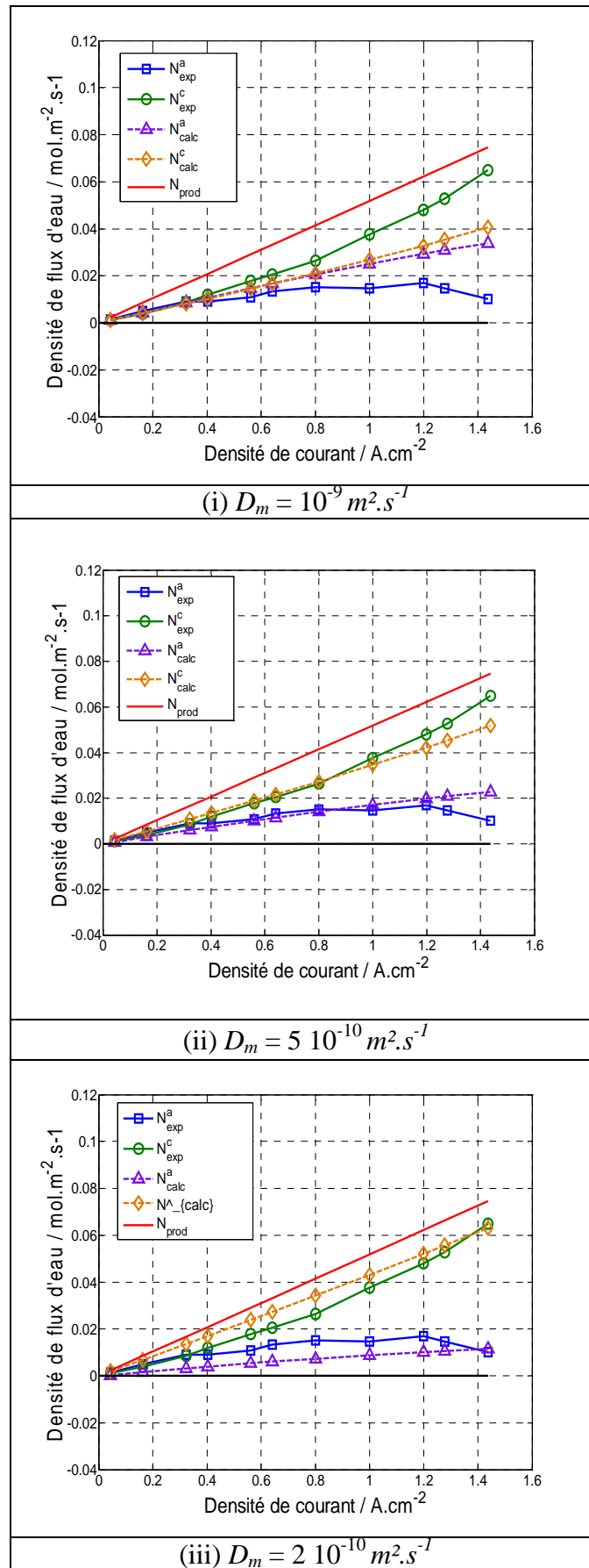
Figure 5.8 Comparaison des densités de flux d'eau calculées et mesurées lorsque T_a = T_c pour D_m = 10^{-9}, 5 \cdot 10^{-10} et 2 \cdot 10^{-10} \text{ m}^2 \cdot \text{s}^{-1} pour \xi = 0
