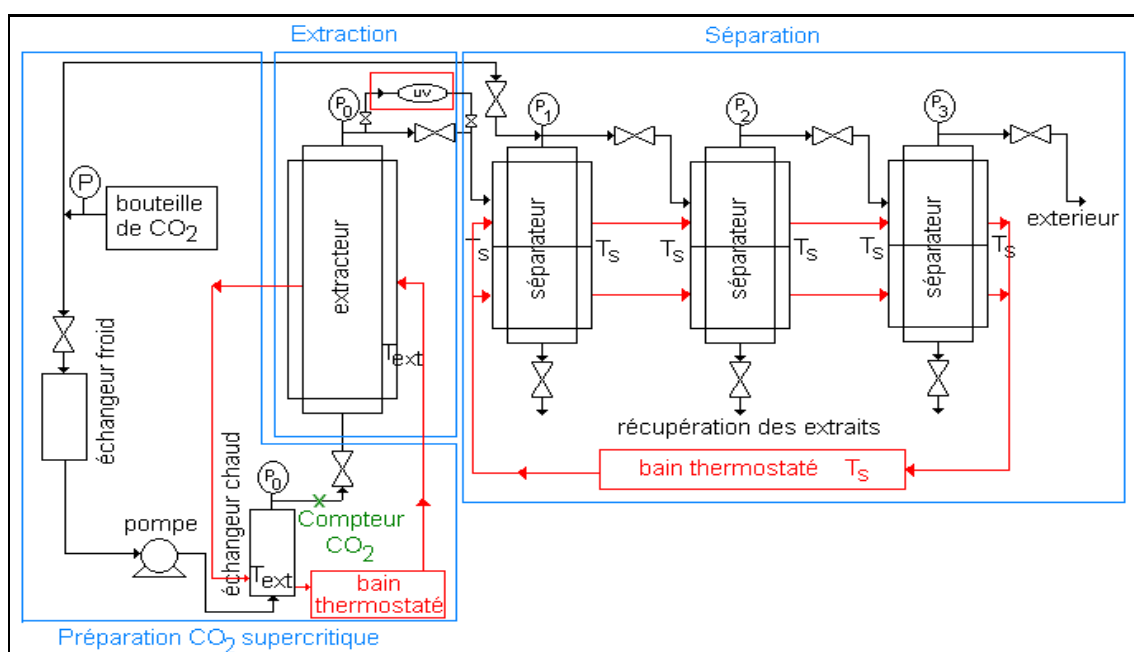
Figure II. 3 Schéma de l'installation d'extraction dynamique ( conditions limites d'utilisations : T = 80\text{ }^{\circ}\text{C} , P = 250\text{ bar} )
