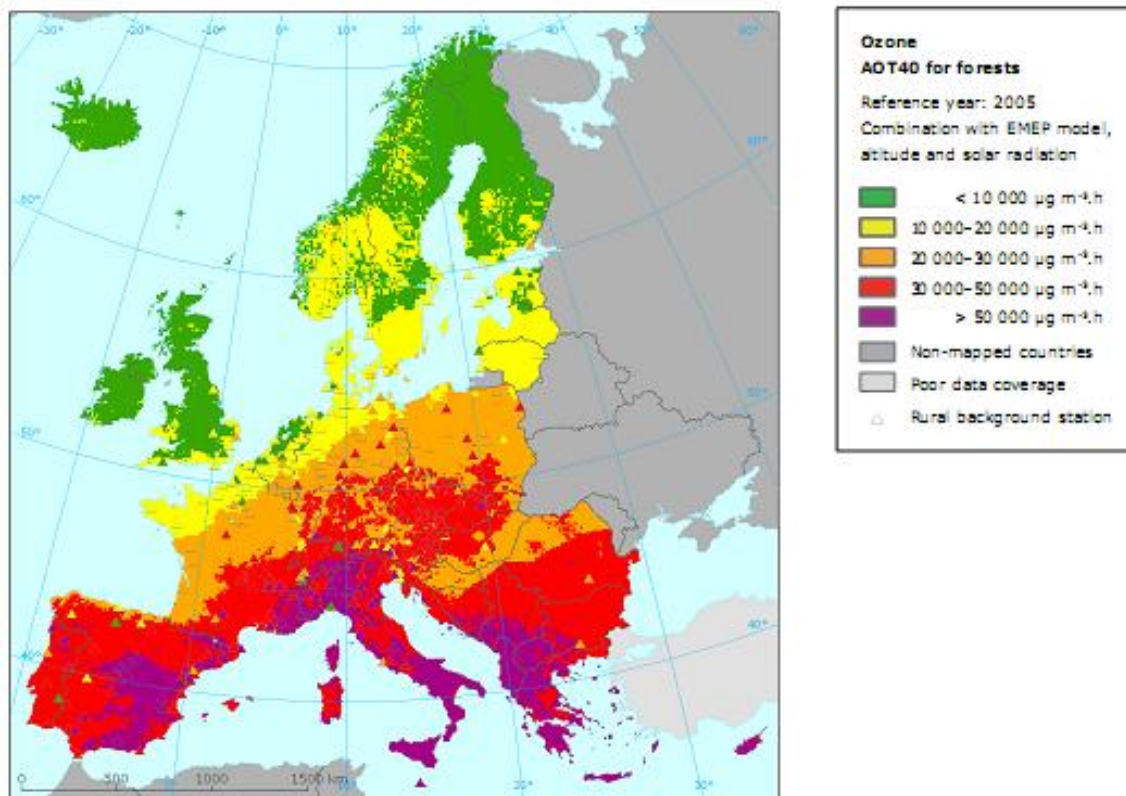
Figure 7 : Cartes des valeurs d'AOT40, indicateur de seuil de risque à l'ozone pour la végétation, en 2005, pour les cultures et pour les forêts (EEA, 2009)
