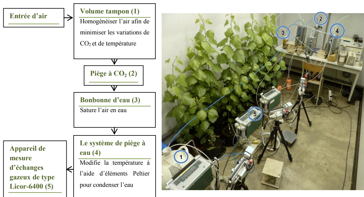
Figure 41 : Schéma du dispositif de mesure avec 3 appareils Li-6400 intercalibrés
