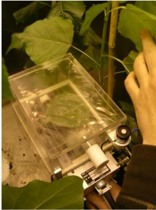
Figure 37 : Mesures réalisées à l'aide de l'appareil de mesure d'échanges gazeux Licor 6200
