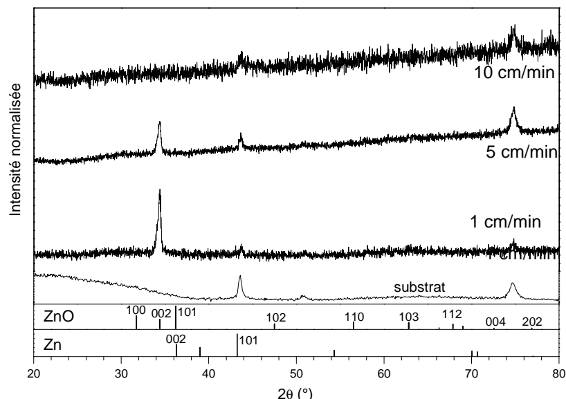
Figure 4-26 : Diffractogramme des dépôts réalisés avec différentes vitesses de défilement.
