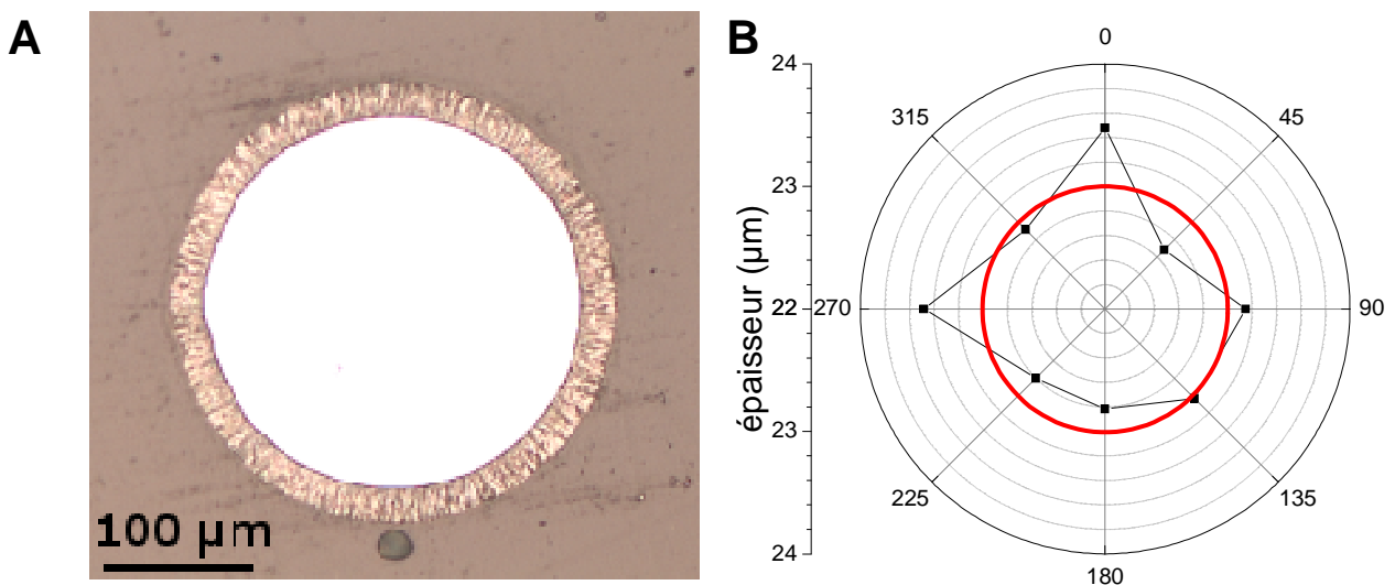
Figure 3-11 : Vue en coupe d'un fil de 250 \mu\text{m} de diamètre recouvert d'une couche de ZnO, grandissement de 20 X (A). Épaisseur du dépôt en fonction de la position circulaire (B). Le cercle rouge représente la moyenne de l'épaisseur. Conditions de dépôt : puissance de 400 W, atmosphère de dépôt est de 2 Pa et est obtenue par l'injection d'un mélange gazeux de 50 % d'oxygène dans l'argon, impulsions de 80 \mu\text{s} , fréquence des impulsions 1 kHz, distance cible-substrat de 8,8 cm, configuration électrique mode c. Vitesse de dépôt de 107 nm/min.
