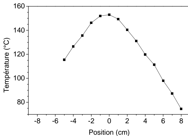
Figure 3-18 : Profil longitudinal de la température du fil pour une puissance moyenne de 400 W en utilisant une durée d'impulsion de 30 \mu s avec une fréquence de 1 kHz et une atmosphère de 2 Pa obtenue par l'injection d'un mélange gazeux de 50 % d'oxygène dans l'argon
