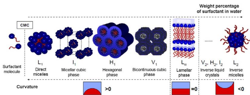
Figure I.1 Différents formes de micelles et phases micellaires. Les parties hydrophobes sont en bleu et les éléments hydrophobes en rouge.
