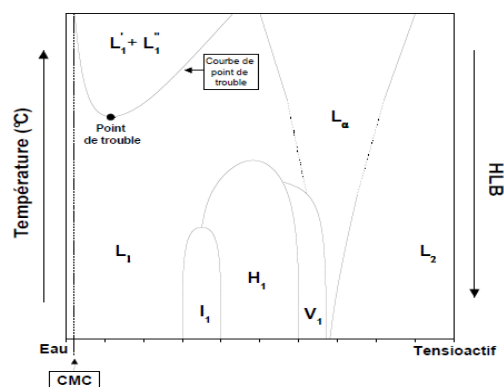
Figure I.2. Diagramme de phase idéal d'un tensioactif.
