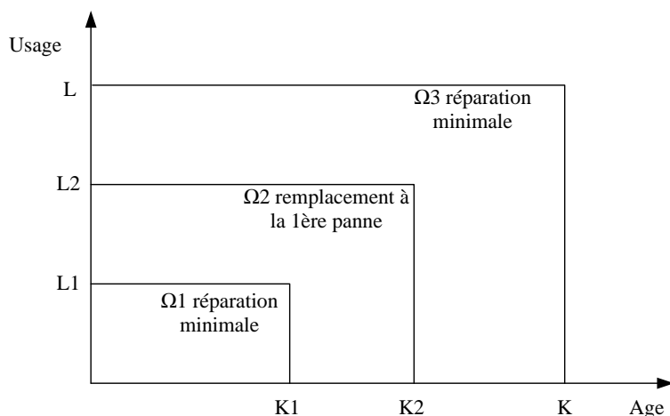
Figure I.15. Stratégie de garantie bidimensionnelle modifiée proposé par (Iskander B.P. et al. (2005))
