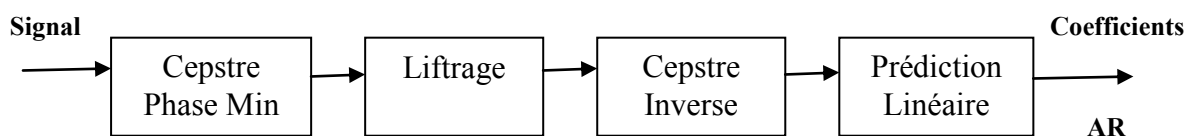
Figure 2. 4 : Diagramme de la méthode prédiction homomorphique proposée par Shahidur (Shahidur Rahman.M 2005)
