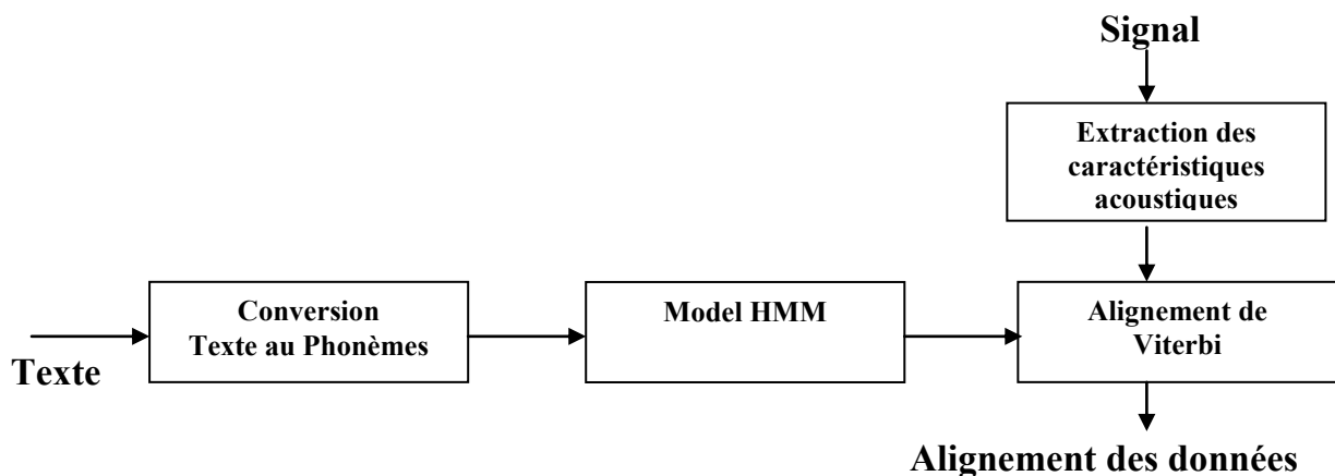
Figure 2. 10 : Schéma de système de segmentation automatique basé sur les HMM (Lee.M 2005)
