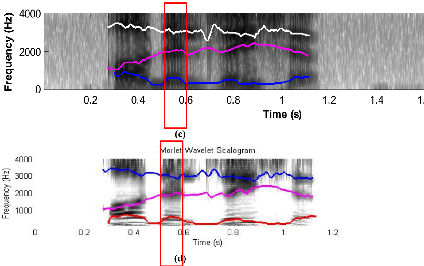
Figure 5. 7 : Trajectoires formantiques estimées du signal sonore « قا:دا لجايشا » « qa:da ljayša » prononcé par la locutrice W4 (a) Etiquetage formantique manuel de référence, (b) Trajectoires formantiques estimées utilisant Praat (c) Trajectoires formantiques estimées utilisant les crêtes de Fourier et (d) Trajectoires formantiques estimées utilisant les crêtes d'ondelette cmor10-1
