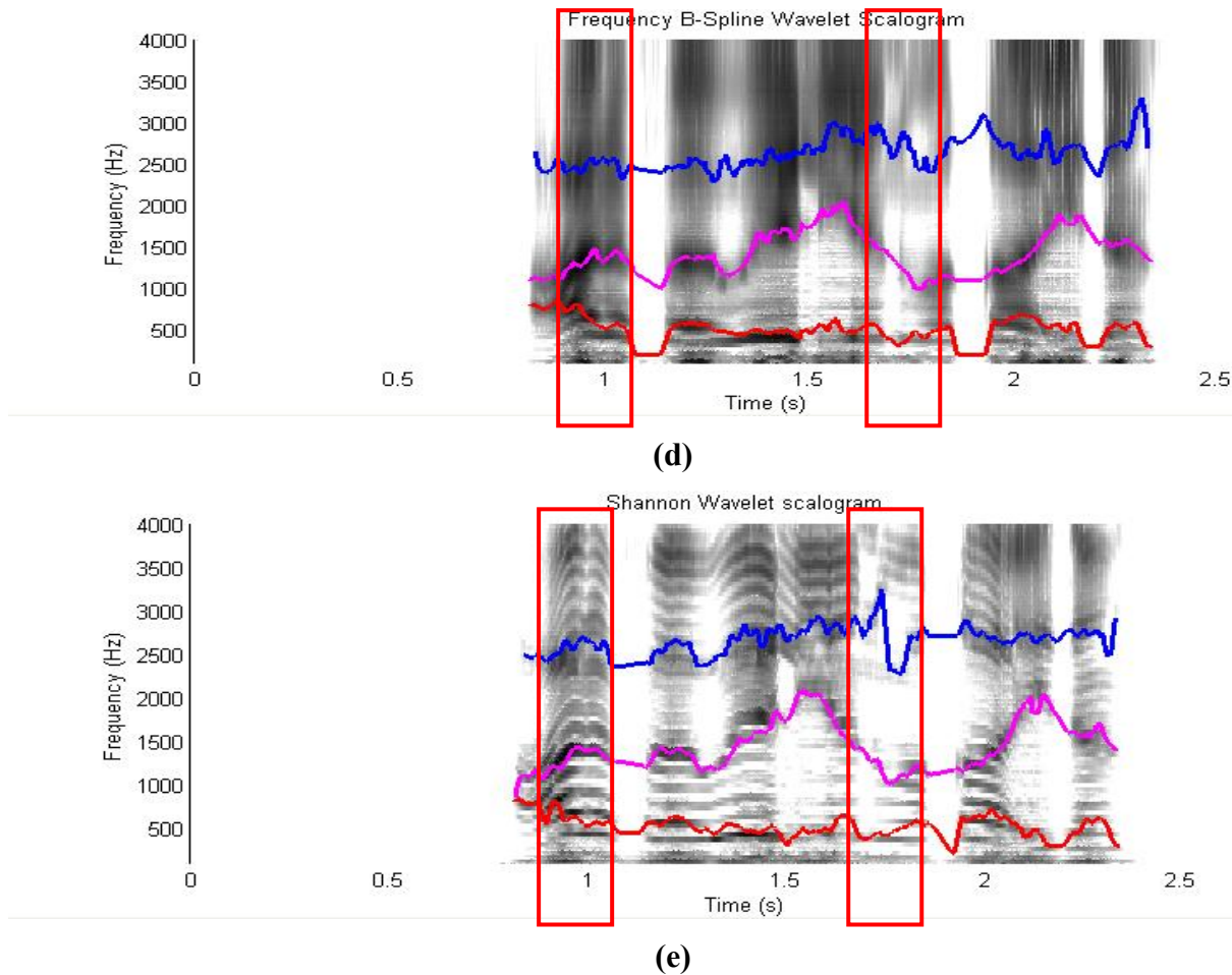
Figure 5. 5 : Trajectoires formantiques estimées du signal sonore « ʿarafa wa:liyan wa qa:3idan » prononcé par le locuteur M1 (a) Etiquetage formantique manuel de référence, (b) Trajectoires formantiques estimées utilisant les crêtes de Fourier et Trajectoires formantiques estimées utilisant les crêtes d'ondelettes : (c) utilisant l'ondelette cmor10-1 , (d) utilisant fbsp10-1-1 , (e) utilisant shan0.1-1 .
