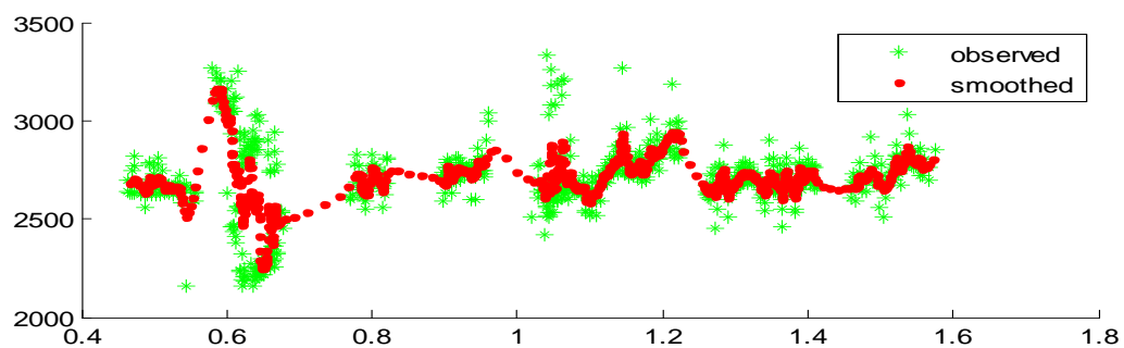
Figure 4.6 : Résultats de filtrage et de lissage de Kalman appliqués sur les trois premiers formants du signal sonore « لَافَاتِي لَانَا:نَا » « zalifati læana:na » prononcée par le locuteur M2 (a) filtrage et lissage de Kalman sur F1, (b) filtrage et lissage de Kalman sur F2, (c) filtrage et lissage de Kalman sur F3.
