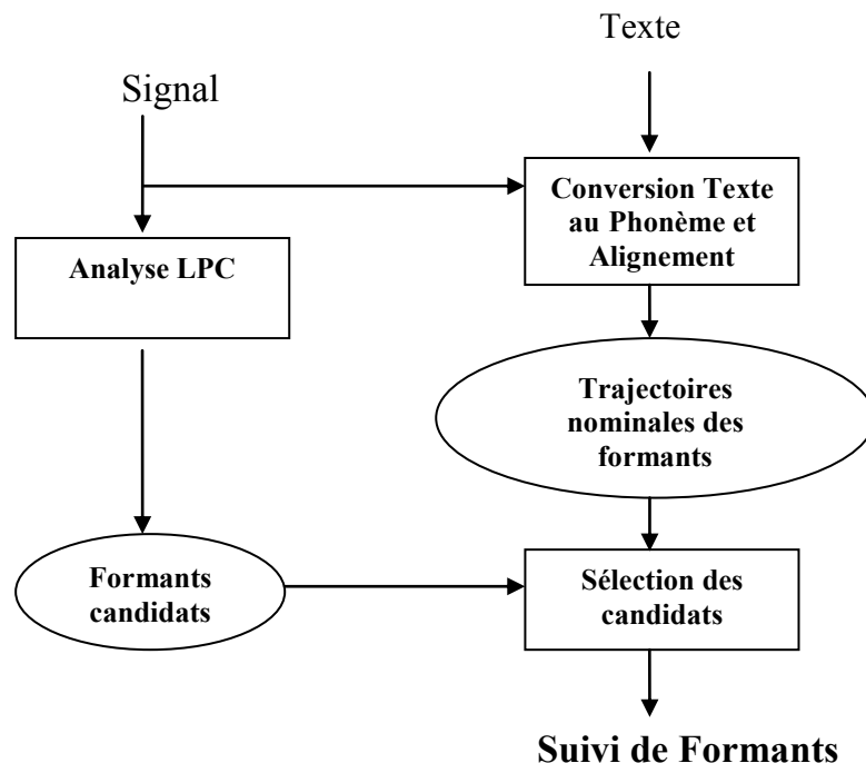
Figure 2. 11 : Schéma global de l'algorithme de suivi de formants proposé par Lee (Lee.M 2005)
