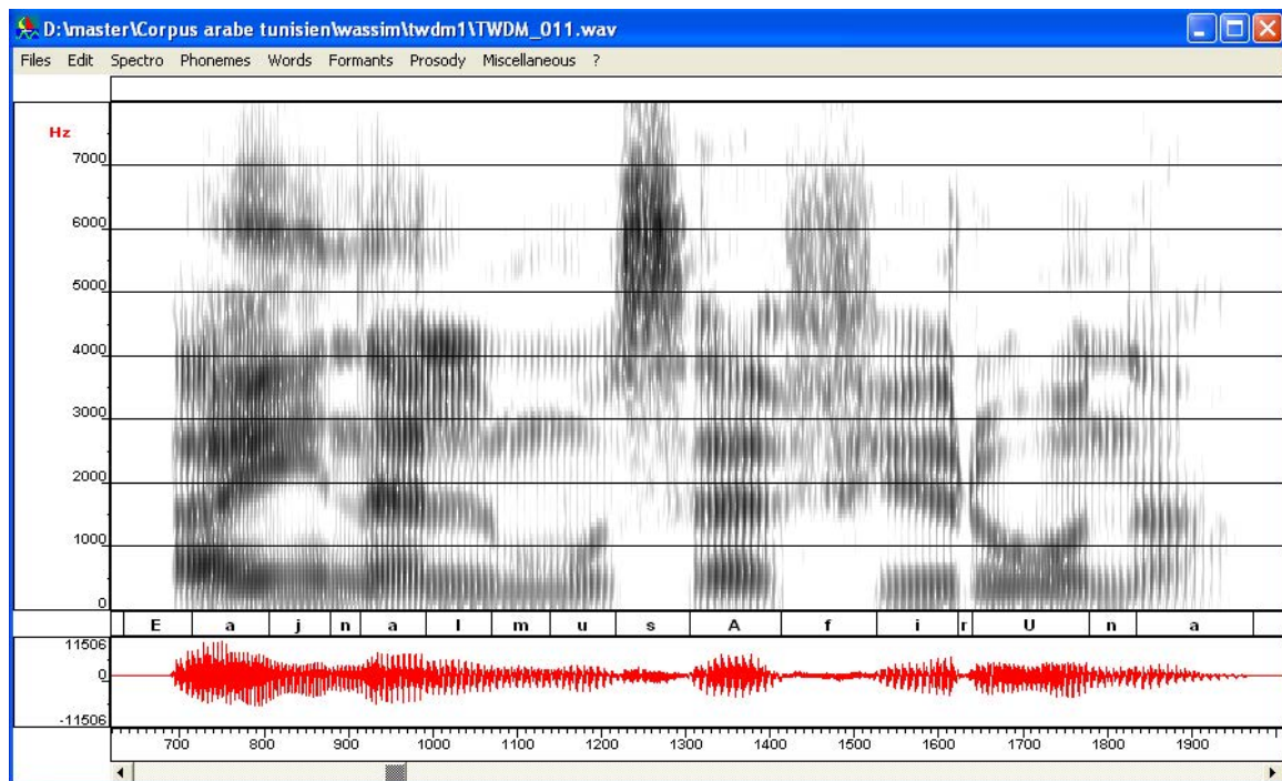
Figure 3. 1 : Spectrogramme de l'enregistrement « يُنَّ لِمُرْفَلِرُونَ ؟ » « 3ayna lmusa:firu:na ? » prononcé par le locuteur Loc.M.4
