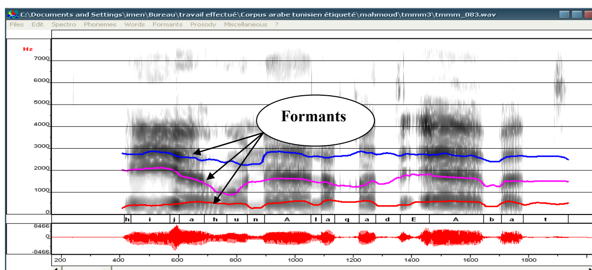
Figure 1.5 : Représentation des trois premiers formants superposés sur le spectrogramme du signal « hiya huna: laqad 3a:bat » « Elle est ici et elle est pieuse »
