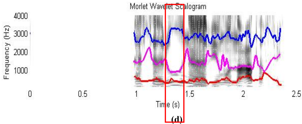
Figure 5. 8 : Trajectoires formantiques estimées du signal sonore « أَوَّلُ » « 3asaru:na: bimunzatafin » prononcé par le locuteur M4 (a) Etiquetage formantique manuel de référence, (b) Trajectoires formantiques estimées utilisant Praat (c) Trajectoires formantiques estimées utilisant les crêtes de Fourier et (d) Trajectoires formantiques estimées utilisant les crêtes d'ondelette cmor10-1
