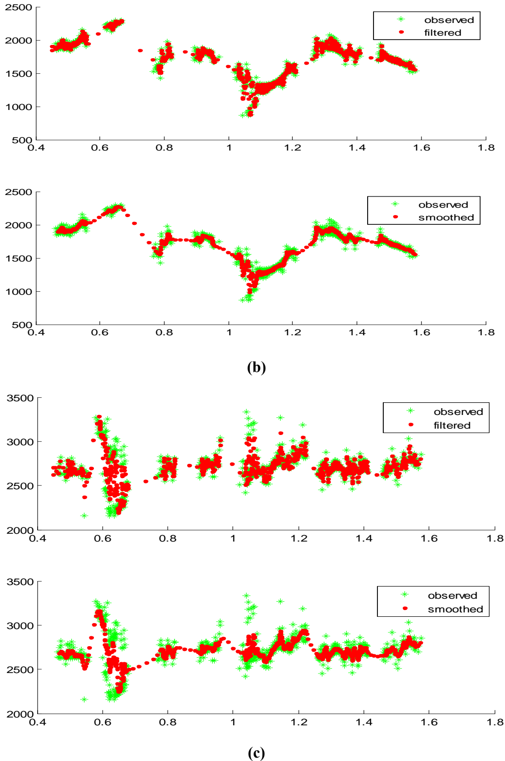
Figure 4.6 : Résultats de filtrage et de lissage de Kalman appliqués sur les trois premiers formants du signal sonore « لَئِيَّ. » « zalifati læana:na » prononcée par le locuteur M2 (a) filtrage et lissage de Kalman sur F1, (b) filtrage et lissage de Kalman sur F2, (c) filtrage et lissage de Kalman sur F3.
