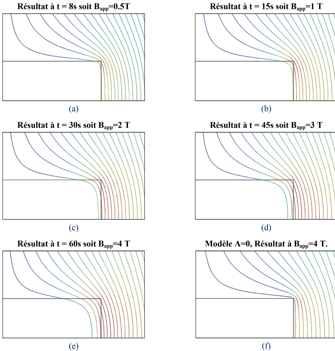
Figure 4.8. Écrantage pour une pastille YBCO \left( J_c = 2 \text{ kA} \cdot \text{mm}^{-2}, n = 30, H_{app} = \frac{4}{(60 \cdot \mu_0)} \cdot t \right) : Lignes de flux autour de la pastille en fonction de B_{app} pour les deux modèles.
