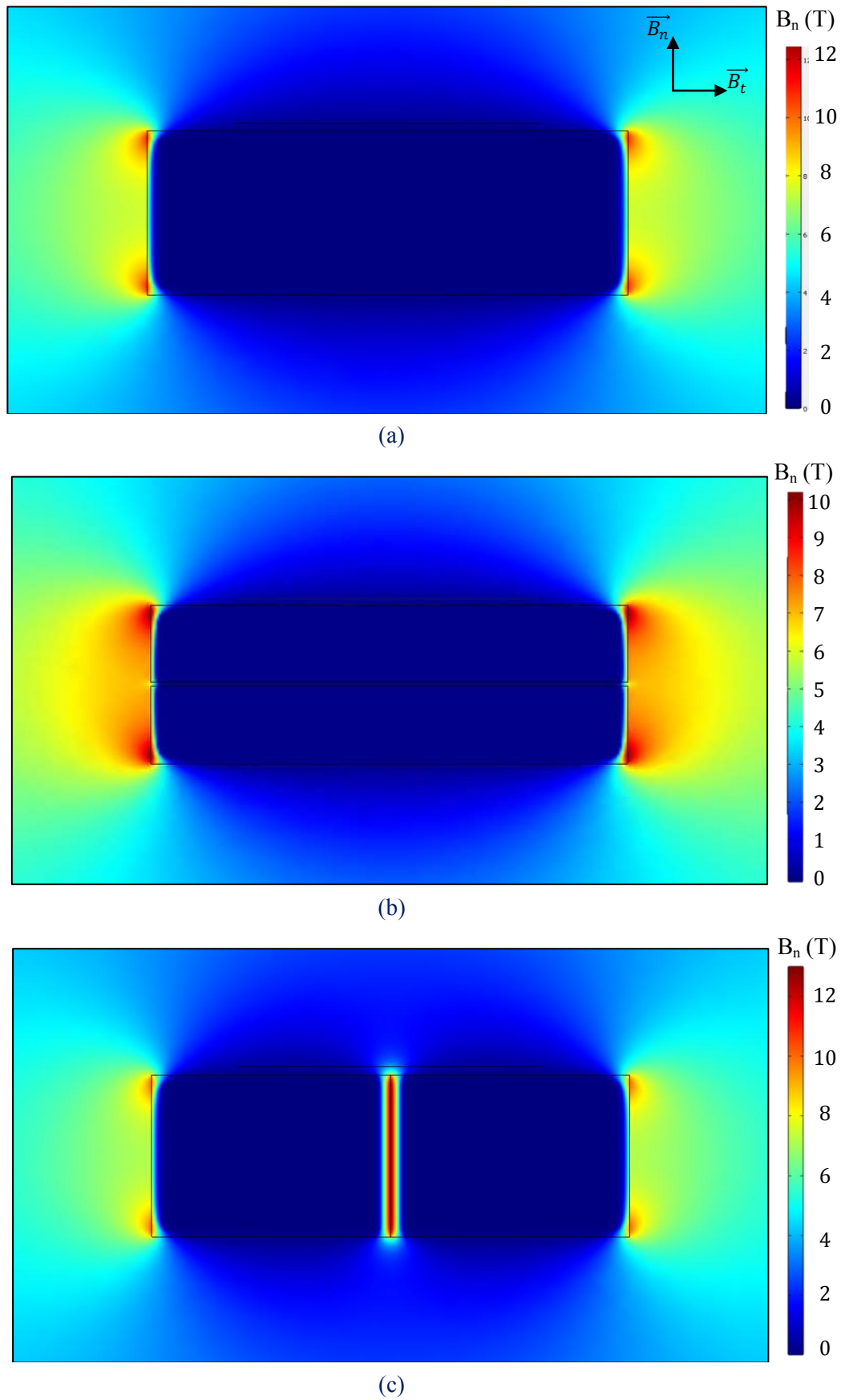
Figure 4.35. Répartition de l'induction magnétique normale ( B_n ) pour \mu_0 H_{app} = 4 \text{ T} : (a) 1P, (b) 2H, (c) 2L.
