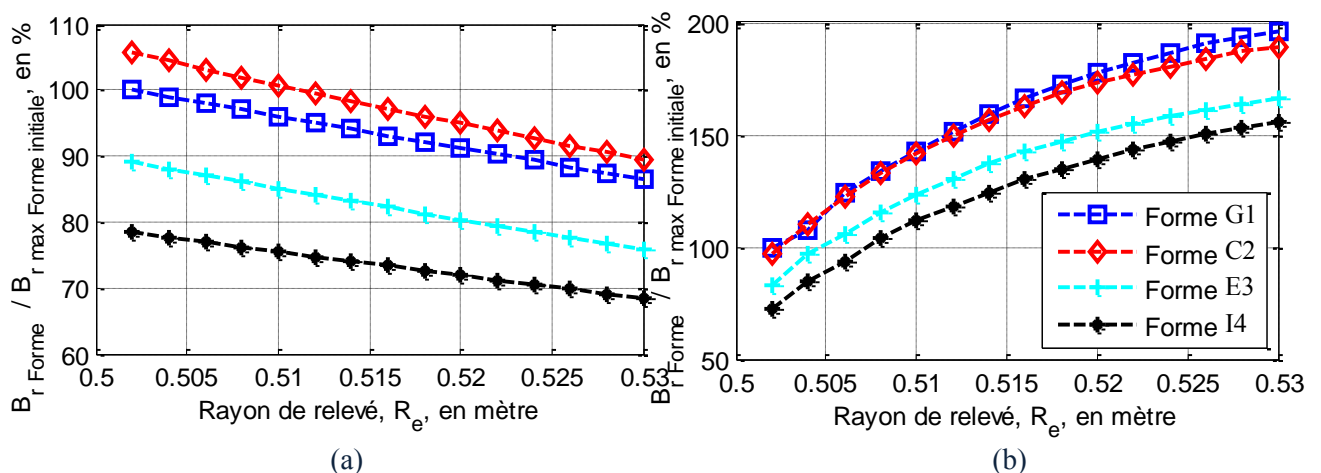
Figure 3.30. Évolution de l'induction radiale moyenne sur la longueur utile (en %) : (a) Entre deux écrans, (b) Derrière un écran.
