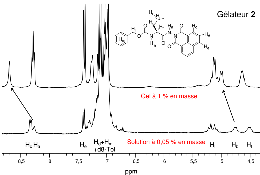
Figure 56 : spectres RMN 1 H à 25°C du gélateur 2 dans le toluène- d 8 en solution à 0,05% en masse et à l'état gel à 1% en masse.
