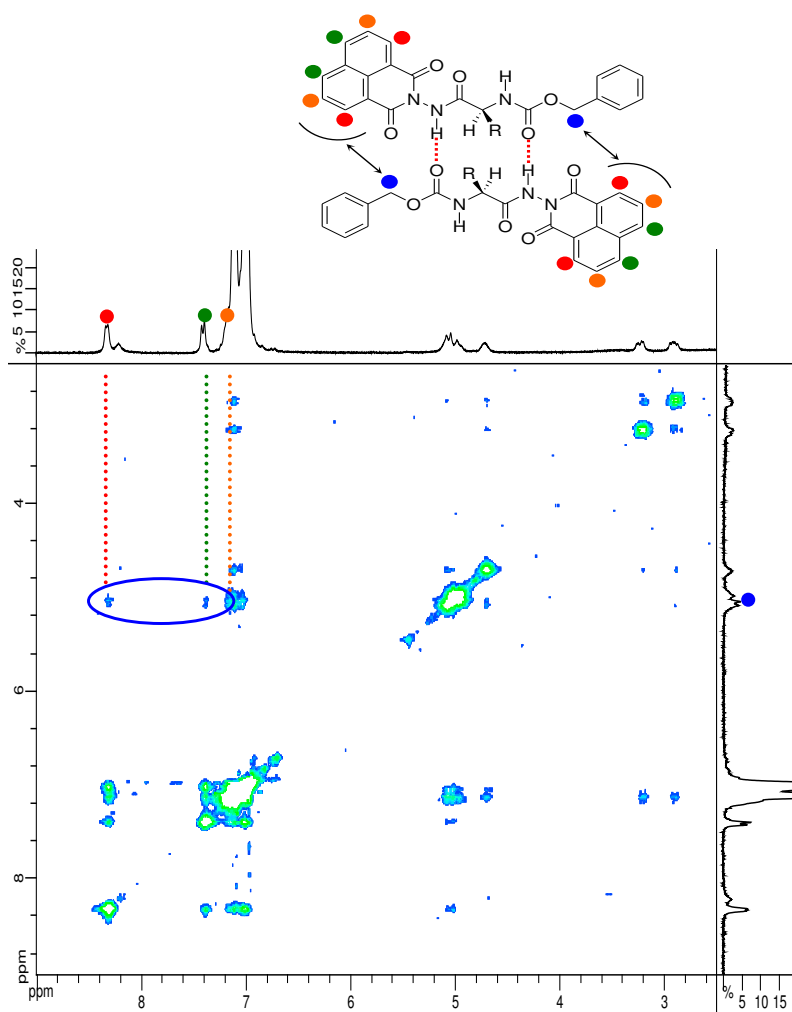
Figure 66 : spectre NOESY du gélateur 1 ( R = \text{CH}_2\text{-Ph} ) à 1% en masse dans le toluène- d 8 obtenu sur un instrument à 300 MHz.
