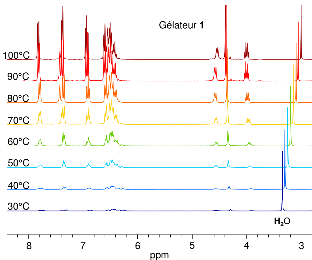
Figure 72 : superposition des spectres RMN 1 H à différentes températures du gélateur 1 à 0,18% en masse dans le tétrachloroéthylène. Le signal des hydrogènes de l'eau présents dans le capillaire de DMSO- d 6, servant d'étalon interne, permet de normaliser l'intensité des signaux des protons du gélateur.
