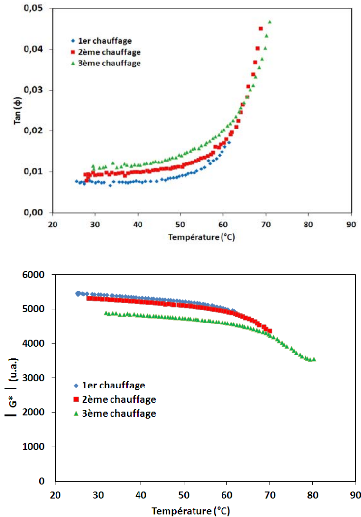
Figure 2-25: Variation du coefficient \tan(\phi) et du module dynamique |G^*| au cours de trois chauffages successifs mesurées à 1 Hz pour le PET des bouteilles de la marque A
