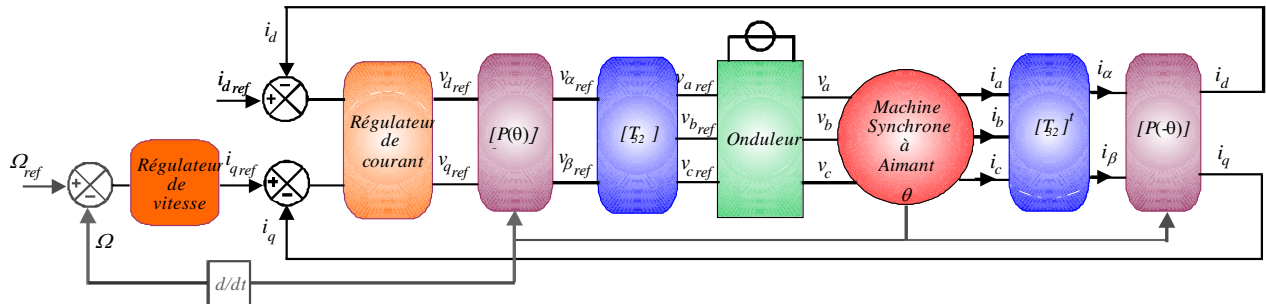
Figure 4-36 : Schéma de régulation en vitesse d'une machine synchrone à aimants alimentée par un onduleur de tension.
