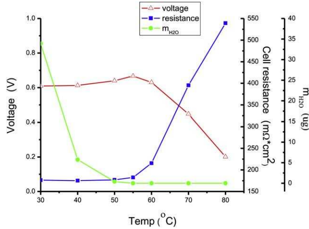
FIG. I.14 – Influence de la température sur les performances de la cellule [ZWFP11] ( i = 0,5 \text{ A.cm}^{-2} , \lambda_{H_2} = 1,2 , \lambda_{H_2} = 2 et HR = 80\% pour les deux gaz).
