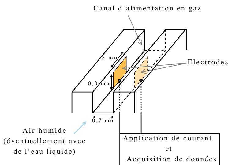
FIG. III.3 – Schéma de principe du montage des électrodes de mesure
