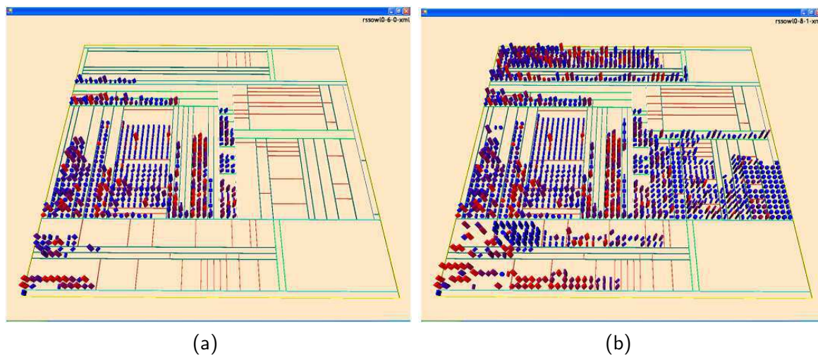
FIGURE 3.29 – Visualisation de l'évolution avec VERSO [LSP08].
