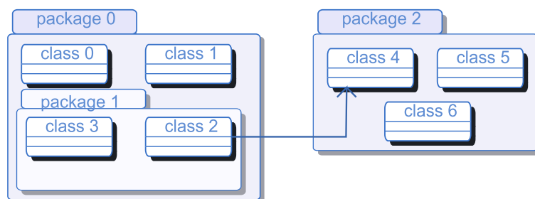
FIGURE 7.1 – Exemple simple de hiérarchie de logiciel.
