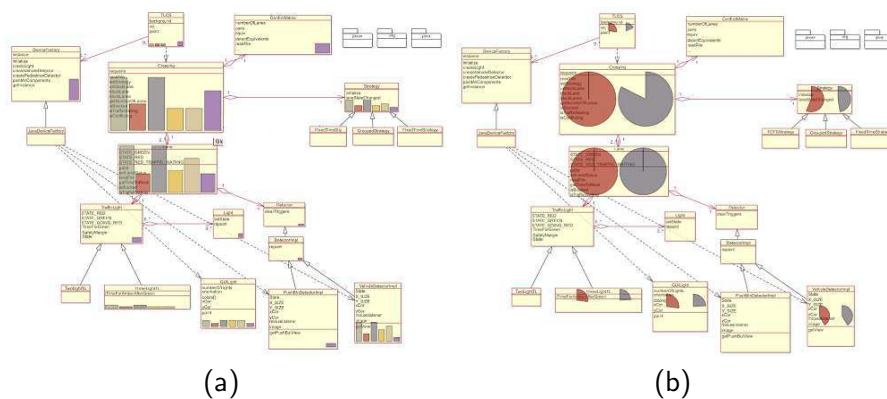
FIGURE 3.18 – (a) MetricView avec diagrammes à barres (b) MetricView avec diagrammes circulaires
