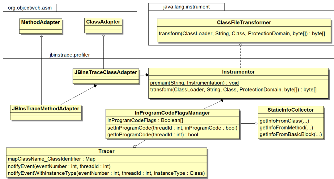
FIGURE 6.6 – Diagramme de classe UML de VITRIL JBinsTrace.
