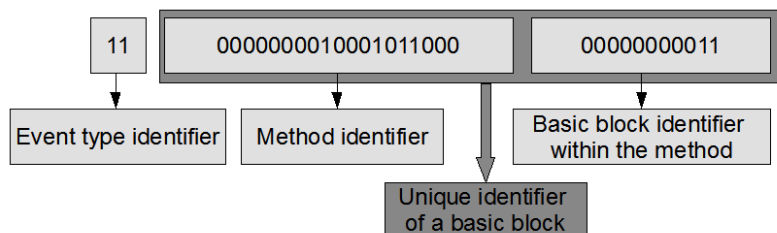
FIGURE 6.3 – Structure de l'entier de 32 bits qui code les événements: « une méthode commence », « une méthode termine », « un bloc de base est exécuté ».
