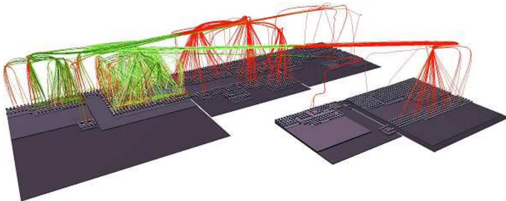
FIGURE 7.11 – Appels dynamique des classes de JEdit. 2710 classes, 2350 arêtes représentant 1 430 347 appels. \beta = 0.8 . Avec courbure des arêtes.
