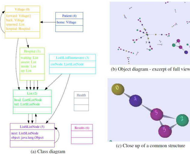
FIGURE 5.8 – Le diagramme de classes et deux visualisations des objets lors de l'exécution de ce programme [MP05].
