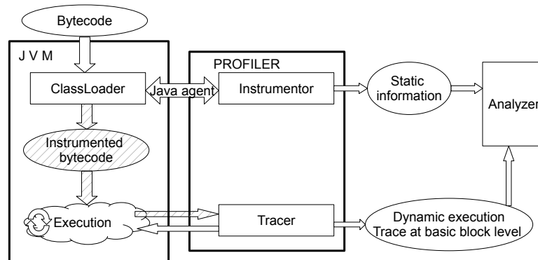
FIGURE 6.1 – Le fonctionnement de notre profileur
