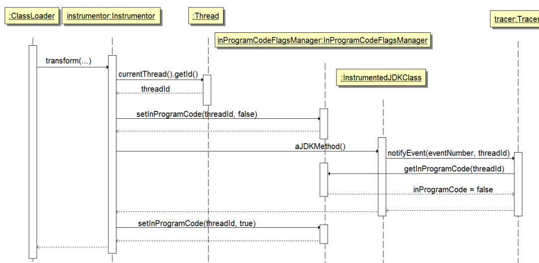
FIGURE 6.5 – Diagramme de séquence montrant les opérations qui permettent d'éviter la pollution de la trace
