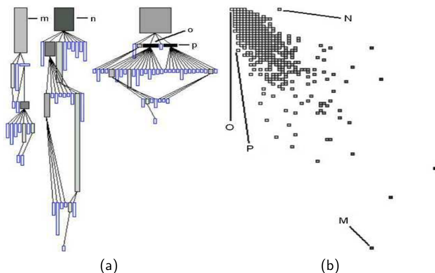
FIGURE 3.20 – Polymetric View [DDL99] : (a) arbre d'héritage et (b) graphe de corrélation.
