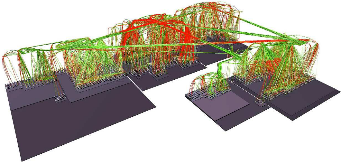
(a) 3D-HEB avec une métaphore de ville utilisant un placement imbriqué
