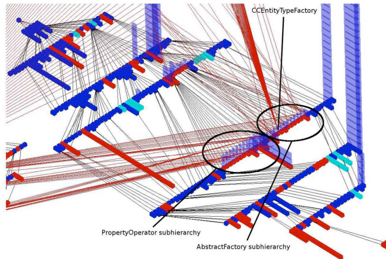
FIGURE 5.7 – Visualisation des relations entre les instances d'un module de Moose[DGN05].
