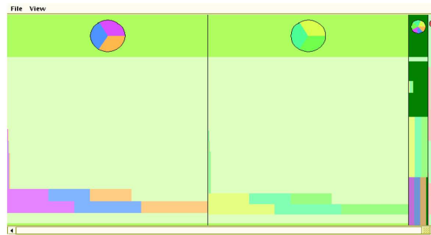
FIGURE 5.2 – Visualisation de l'exécution d'un programme Java avec JOVE [RR05].
