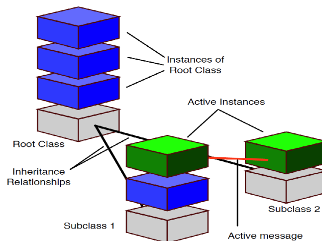
FIGURE 5.6 – Une vue schématique de la vue polymétrique en 3D [GLW05].
