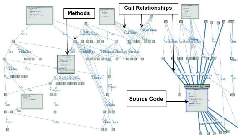
FIGURE 3.11 – Visualisation du graphe d'appel avec l'outil SHriMP.
