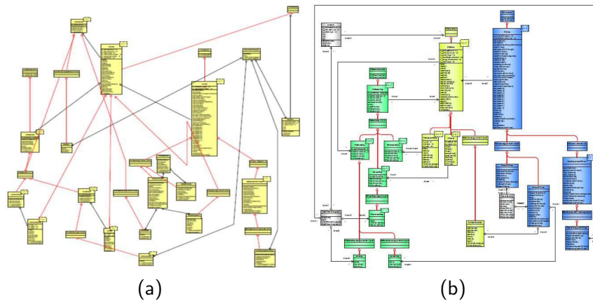
FIGURE 3.9 – (a) Placement classique. (b) Le placement de GoVisual [GJK + 03].
