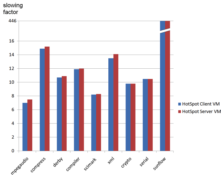
FIGURE 6.7 – Résultats de performance sur les tests de performances SPECjvm2008.
