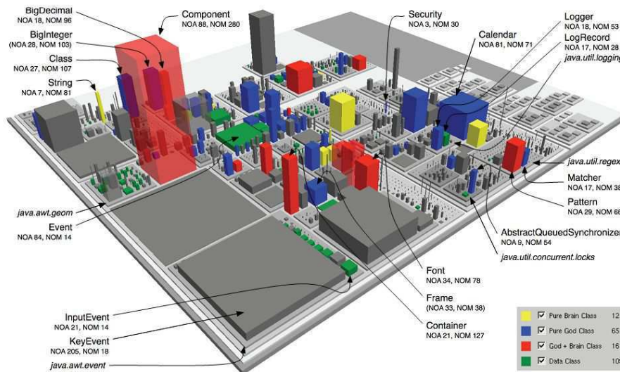
FIGURE 3.23 – Carte des problèmes de conception avec CodeCity [WL08b].
