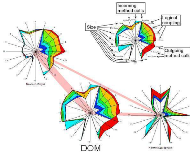
(a) Métriques sur les modules
