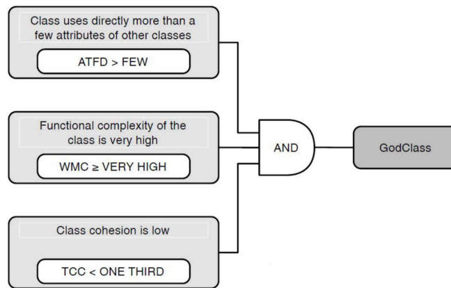
FIGURE 2.2 – Détection d’une classe God [LM06]
