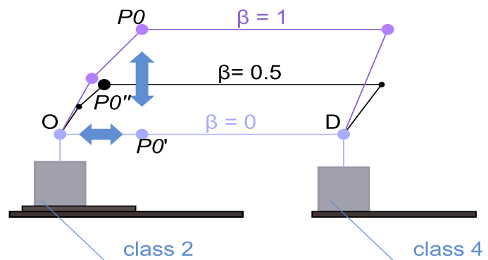
FIGURE 7.8 – Interpolation des P_n en fonction du facteur \beta .
