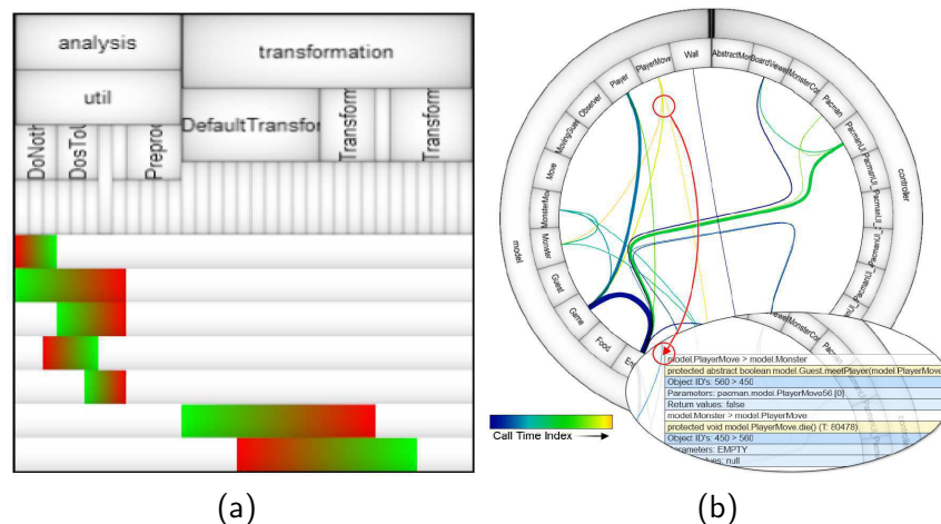
FIGURE 5.5 – (a) Massive Sequence, (b) HEBs avec vue temporelle [HCvW07a, CHZ + 07].
