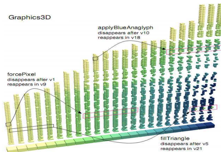
FIGURE 3.26 – Timeline [WL08a] pour visualiser l'évolution de la classe : Graphics3D du logiciel Jmol
