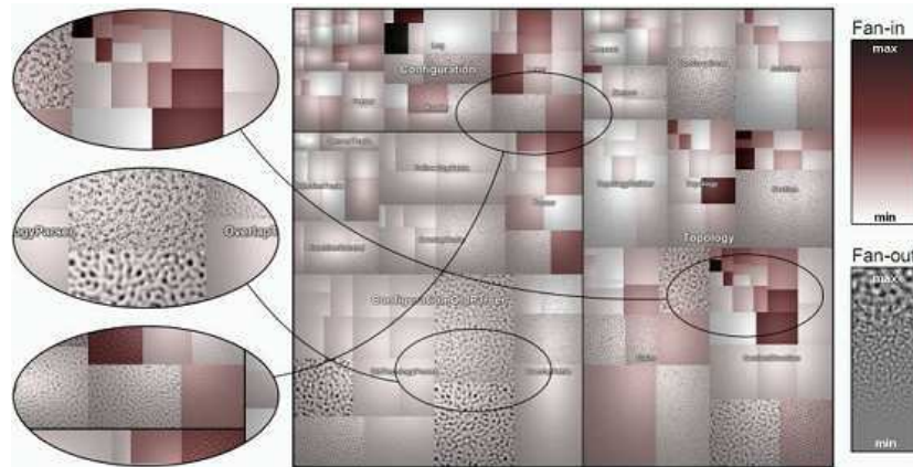
FIGURE 3.21 – Treemap avec couleurs et textures [HVvW05].
