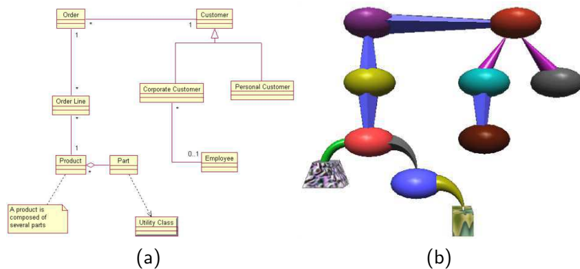
FIGURE 3.10 – (a) UML diagramme (b) le diagramme de Geon équivalent.
