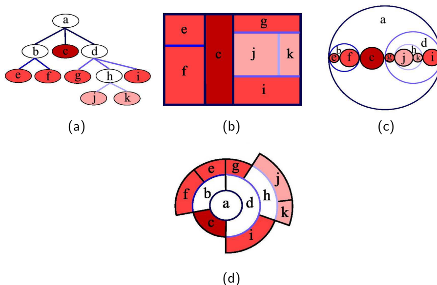
FIGURE 3.3 – (a) Node-Link diagrams (b) Treemap (c) Circular Treemap (d) Sunburst. Toutes ces figures représentent le même système.
