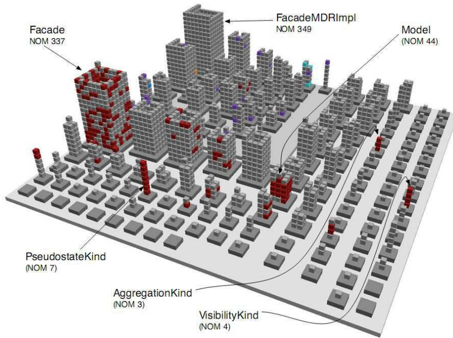
FIGURE 3.24 – La carte des problèmes de conception avec CodeCity au niveau de la méthode[WL08b].
