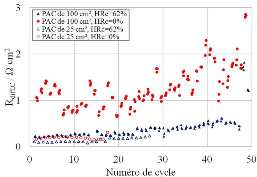
FIGURE III.29 – Résistance de diffusion cathodique R_{diff,C} au cours du cyclage à faible HR (62%/0%) réalisé sur la pile de 25 cm 2 et sur celle de 100 cm 2 .
