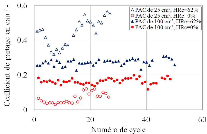
FIGURE III.26 – Coefficient de partage en eau au cours du cyclage à faible HR (62%/0%) réalisé sur la pile de 25 \text{ cm}^2 et sur celle de 100 \text{ cm}^2 .
