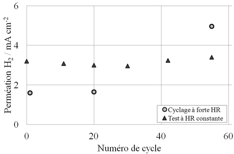
FIGURE III.7 – Densité de courant correspondant à la perméation de l’hydrogène au cours du cyclage à forte HR (62%/100%) et du test à HR constante.
