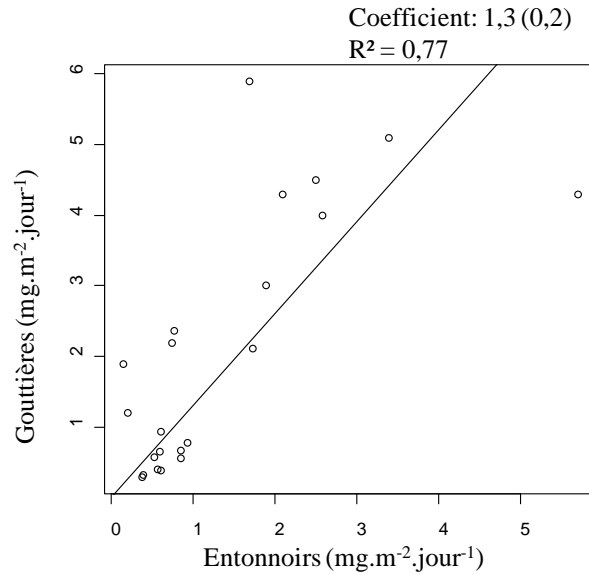
Figure 26 : Inter-comparaison des 2 types de collecteurs, entonnoirs et gouttières, à partir des taux de dépôts H-ADD en \text{mg.m}^{-2}.\text{jour}^{-1} dans le site de Montiers entre décembre 2010 et mars 2011, et juin 2011 et mars 2012.
