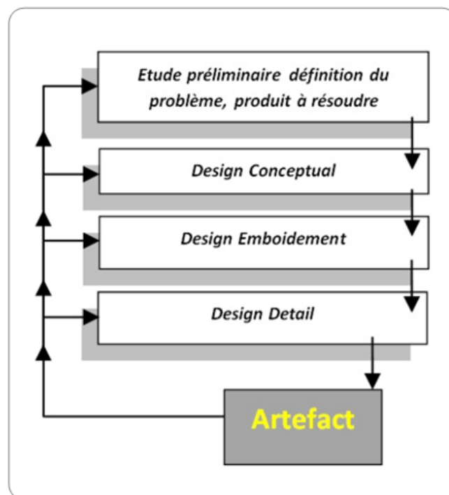
Figure 30 : Le modèle du processus de conception. Pahl & Beitz 1977. Source : (Pialot, 2009)
