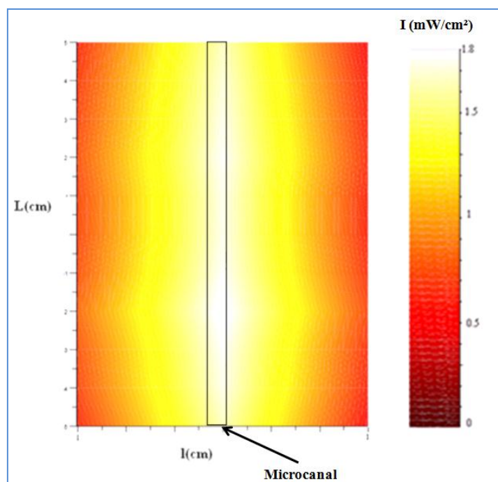
Figure II. 13 : Distribution de la lumière dans un plan à une distance L_d = 10 cm de la lampe UV.
