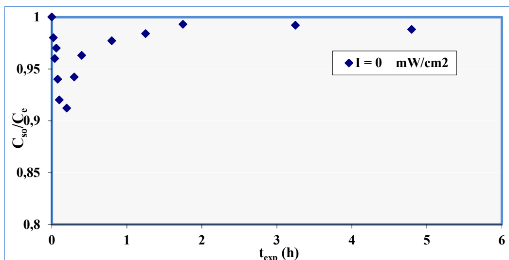
Figure III.2 : Variation de C_{so}/C_e en fonction du temps d'expérience dans Rinox, à un débit de 5 mL/h, en absence d'irradiation ; C_e = 10 \text{ mg/L} .
