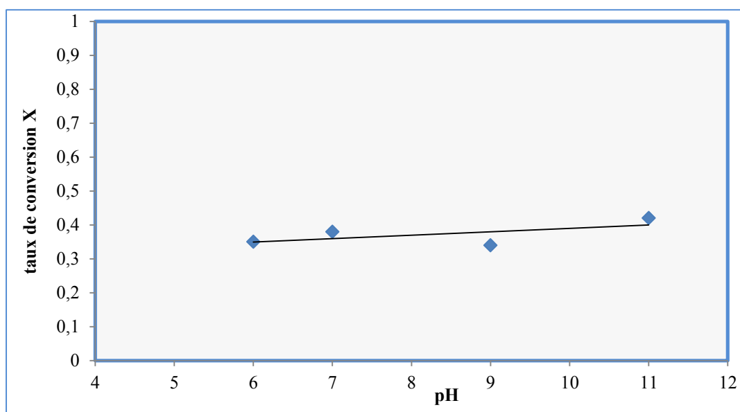
Figure III.18 : Variation du taux de conversion en fonction du pH, dans le microréacteur R4, Q = 2,5 \text{ mL/h} , C_e = 10 \text{ mg/L} et I = 1,5 \text{ mW/cm}^2 .
