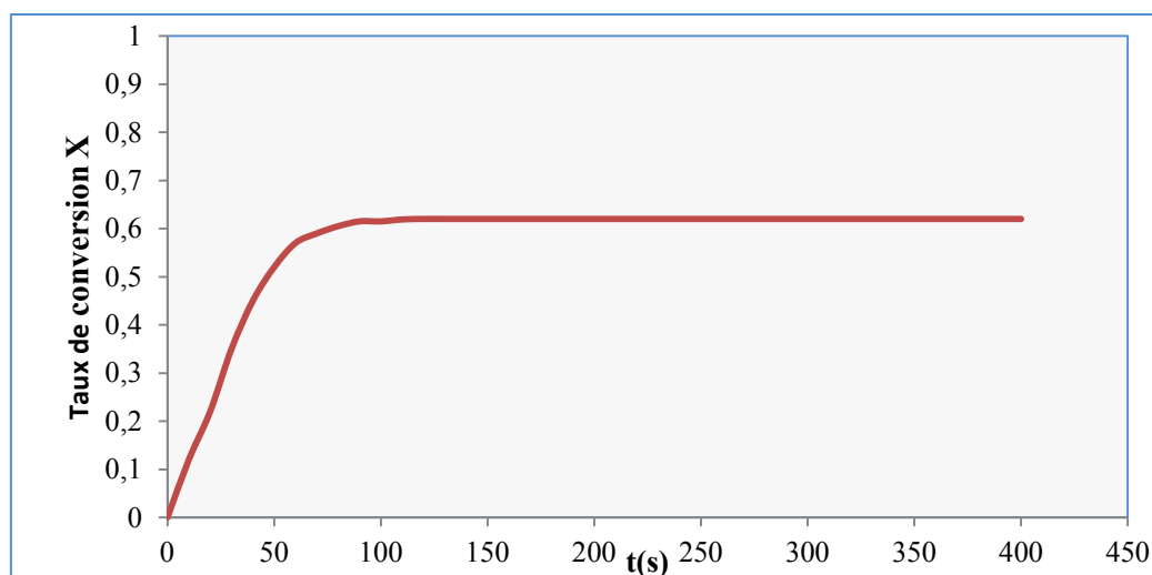
Figure V. 5 : Variation du taux de conversion en fonction du temps de simulation dans le microréacteur R1, Q = 2,5 \text{ mL/h} et C_e = 10 \text{ mg/L} .
