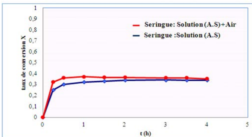
Figure III.19: Variation du taux de conversion en fonction de la présence d'oxygène, dans le microréacteur R4, Q=2,5 mL/h, C_e=10 mg/L et I = 1,5 mW/cm 2 .
