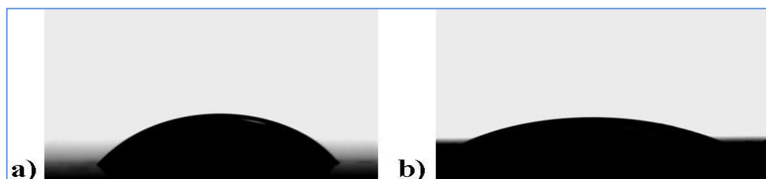
Figure II. 9 : Influence de l'éthanol sur l'étalement de la suspension de \text{TiO}_2 à la surface du polymère : a) Suspension aqueuse ; b) Suspension avec 30 % volumique d'éthanol.
