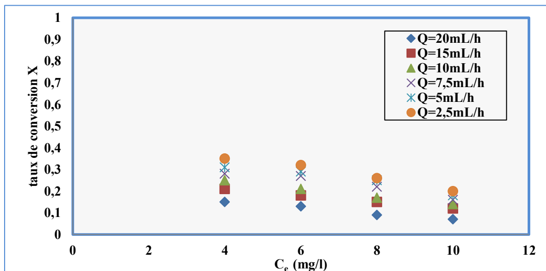
Figure III.15 : Variation du taux de conversion en fonction de la concentration d'entrée C_e , dans le microréacteur Rinox, pour différents débit et pour I = 1,5 \text{ mW/cm}^2 .
