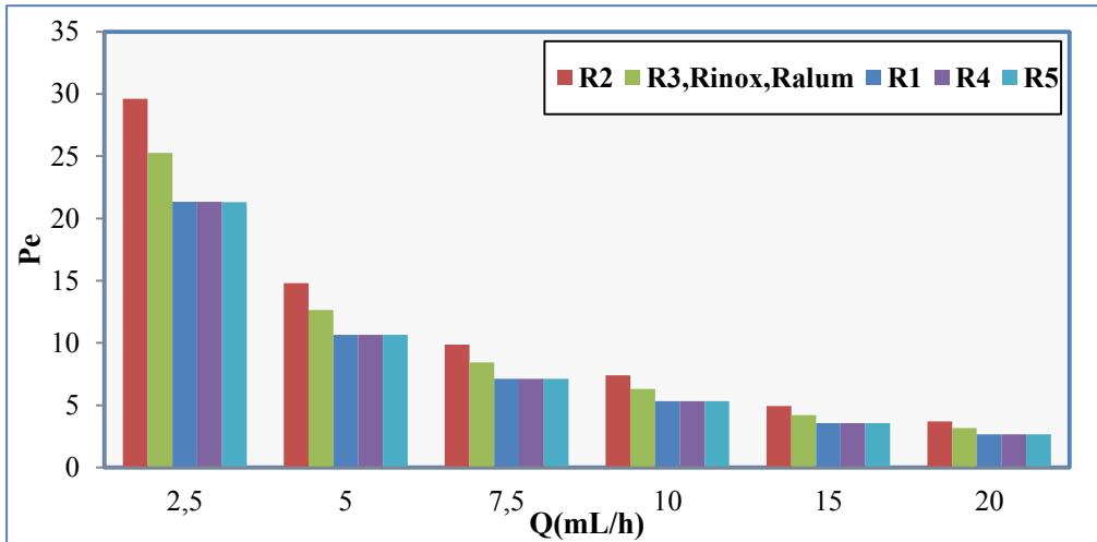
Figure III.29 : Nombre de Péclet calculé par la relation en fonction du débit pour les différents microcanaux.
