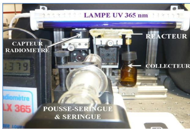
Figure III.1 : Photo du montage expérimental (Charles et al., 2011).
