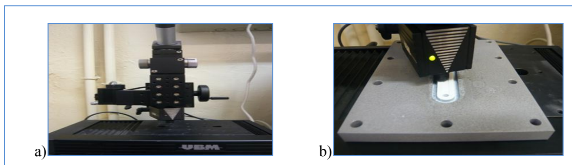
Figure II. 10 : Photographie du profilomètre avec : a) vue d'ensemble, b) détail de la tête de mesure équipée d'une lentille dynamique de focalisation à la surface de l'échantillon.
