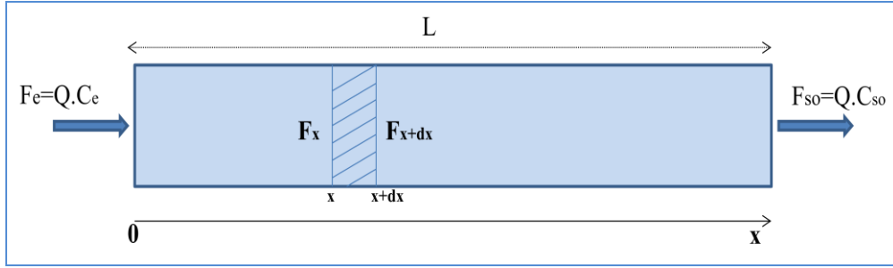
Figure III.25 : Schéma représentatif d'un réacteur piston parfait.
