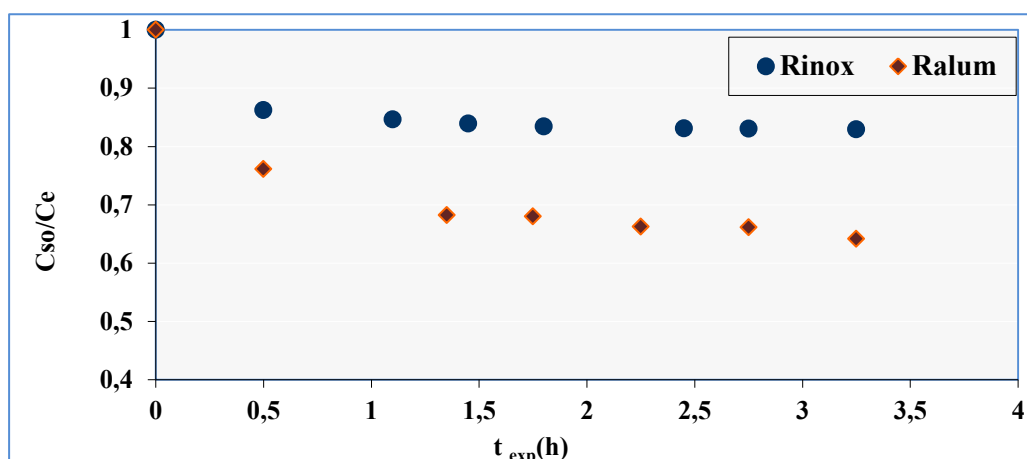
Figure III.22 : Variation de la concentration relative Cs en fonction du temps dans les microréacteurs Rinox et Ralum ; I = 1,5 mW/cm 2 , C e = 10 mg/L et Q = 5 mL/h.
