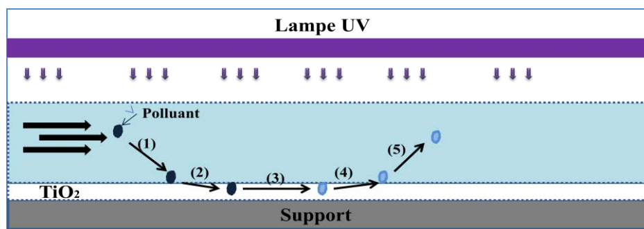
Figure III.24 : Schéma représentatif du processus réactionnel.
