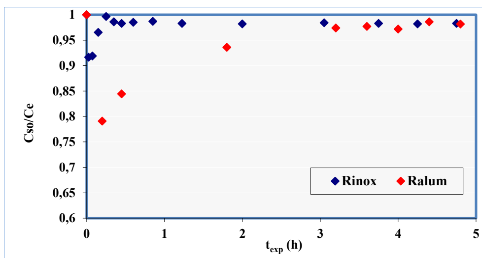
Figure III.20: Variation de la concentration relative de sortie C_{so} en fonction du temps d'expérience dans les microréacteurs en inox et en aluminium ; I=0 \text{ mW/cm}^2 , C_e = 10 \text{ mg/L} et Q = 2,5 \text{ mL/h} .
