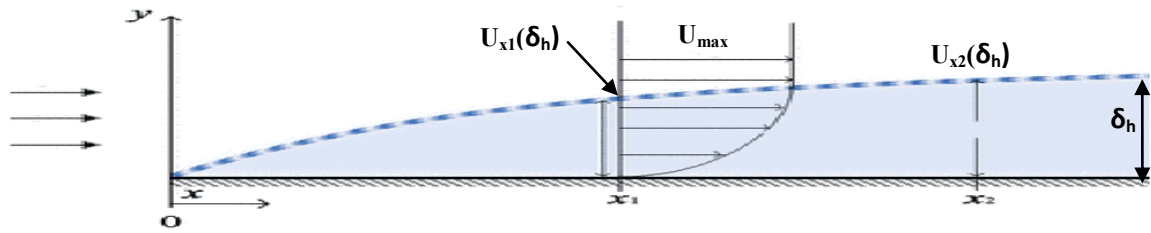
Figure IV. 12: Variation de la vitesse d'écoulement au travers d'une couche limite au dessus d'une plaque plane.
