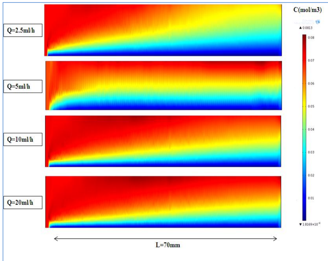
Figure V. 6 : Gradient de la concentration en fonction du débit d'entrée dans le microréacteur R1 avec C_e = 10\text{ mg/L} .
