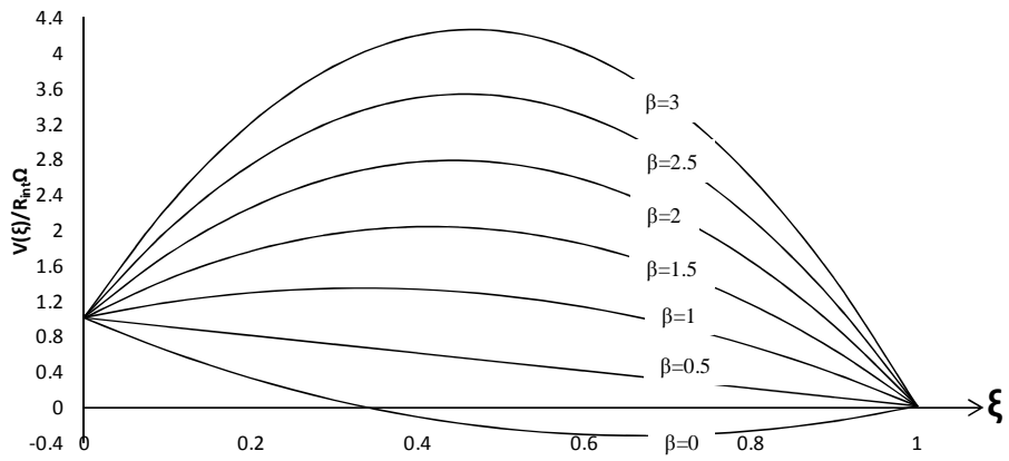
Figure 16 : Profils de vitesses des écoulements obtenus par variation du rapport de vitesse débitante sur vitesse de rotation du cylindre interne dans le réacteur Couette-Poiseuille ( \beta ).
