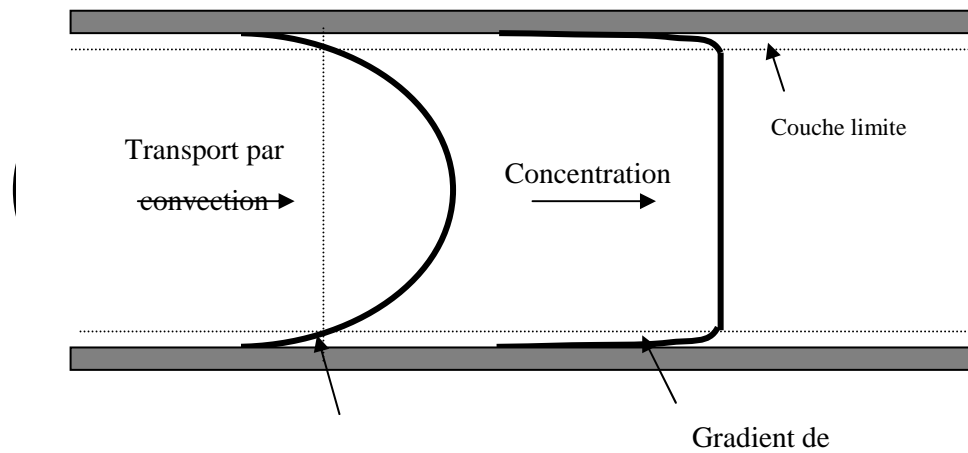
Figure 5 : Représentation schématique des processus de transport dans une chambre d'écoulement.
