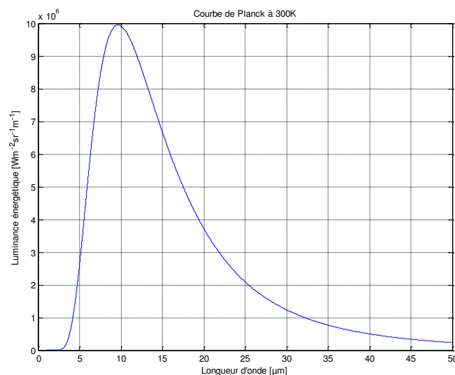
Figure IV.22 : Spectre de luminance énergétique d'un corps noir à 300 K (courbe de Planck).
