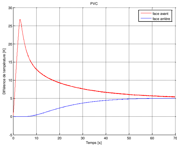
Thermogrammes expérimentaux
