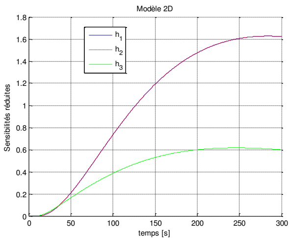
Modèle bidirectionnel à flux connu
