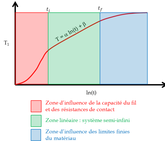
Figure II.8 : Illustration des limites de la zone linéaire de la température du fil chaud.
