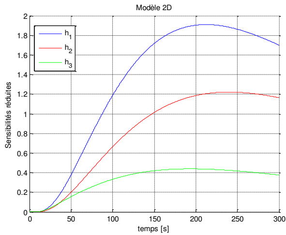
Modèle bidirectionnel dépendant du flux
