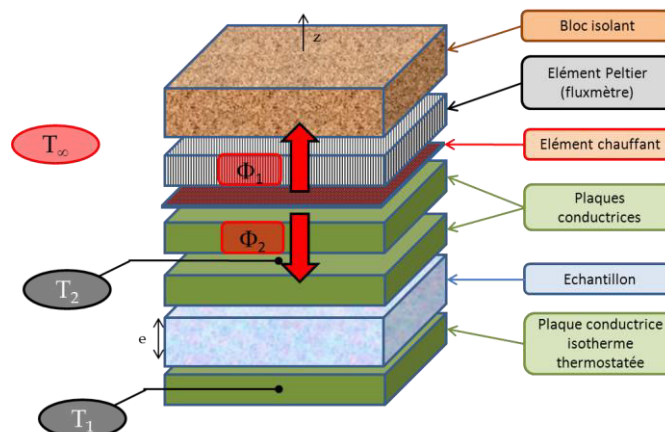
Figure II.6 : Schéma de principe de la méthode de la mini-plaque chaude.
