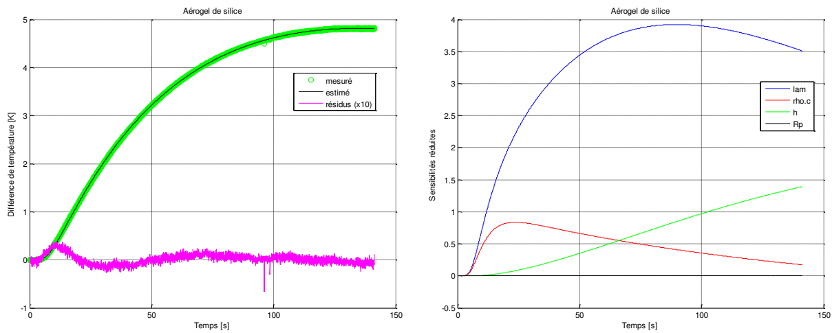
Thermogrammes de la face arrière
