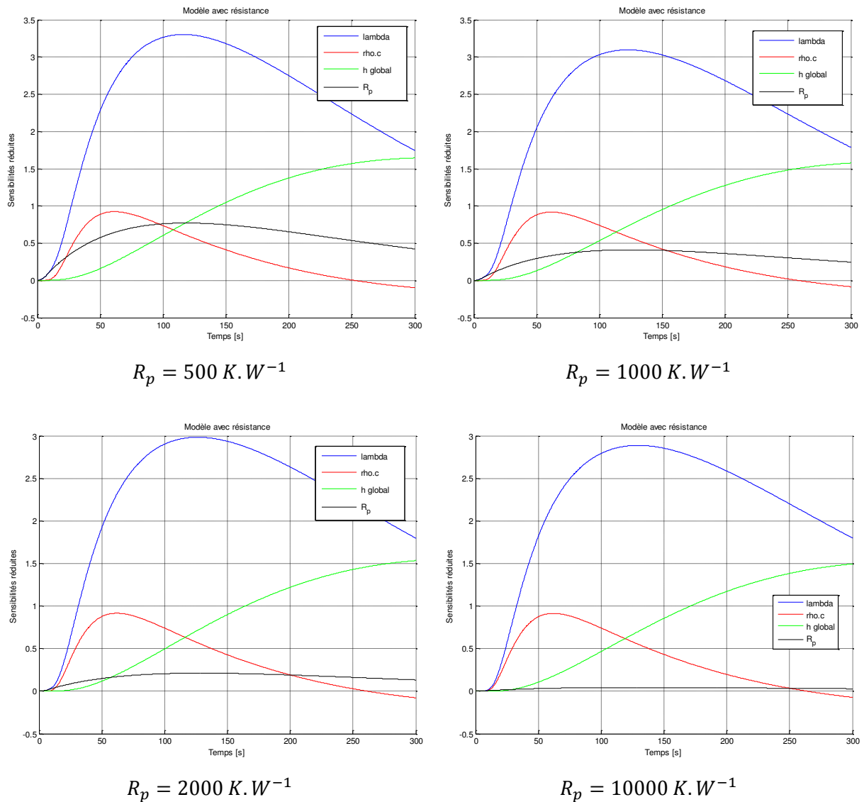
Figure III.18 : Sensibilités réduites du modèle avec prise en compte de la résistance en parallèle.
