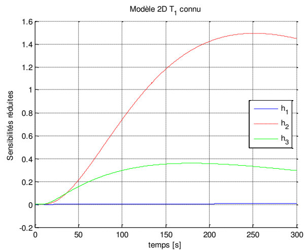
Modèle bidirectionnel dépendant de la température de la face avant
