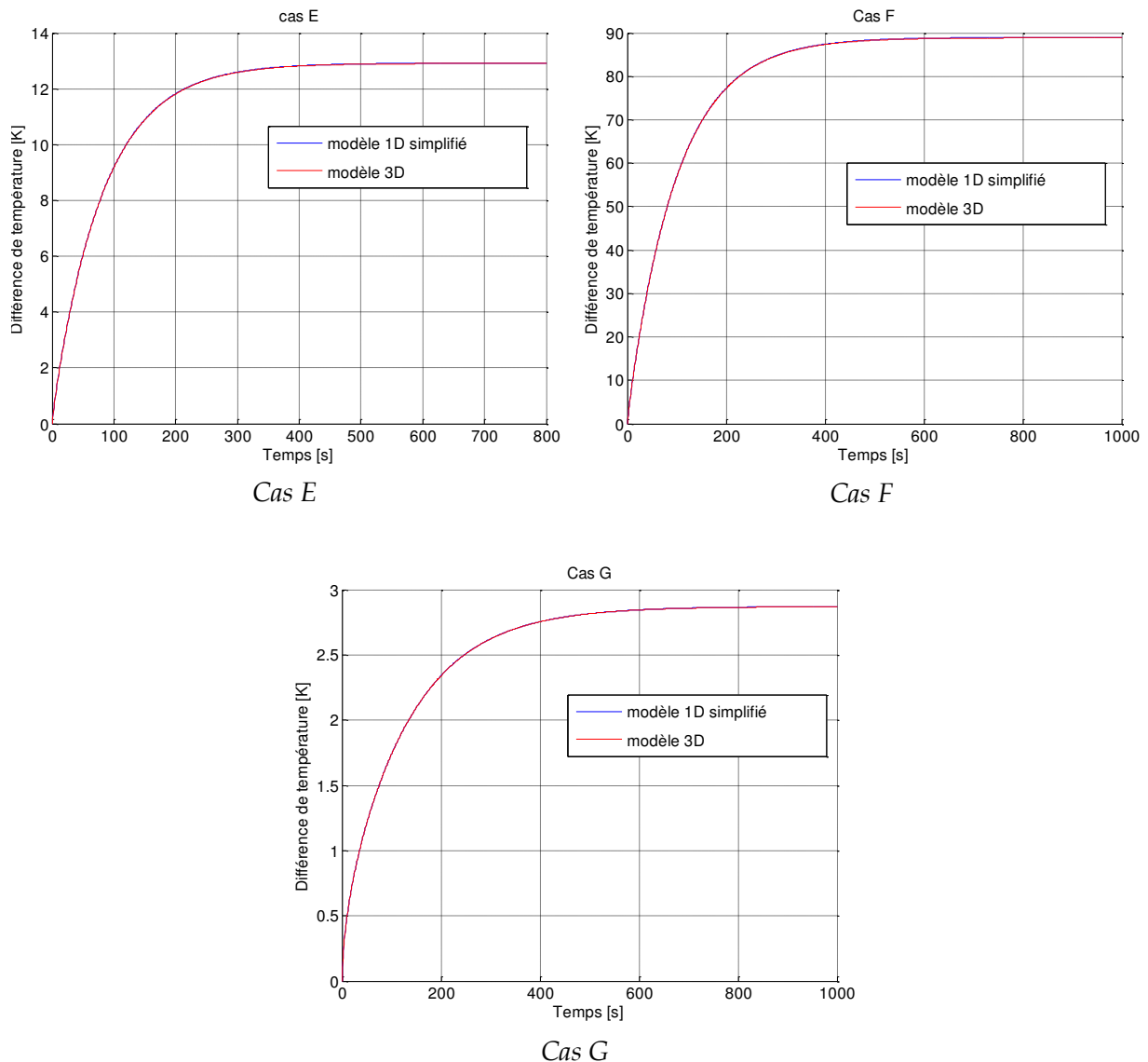
Figure IV.27 : Comparaison du modèle unidirectionnel simplifié avec le modèle à trois dimensions.
