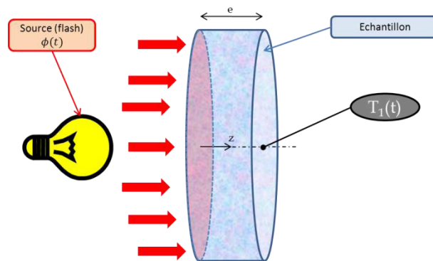
Figure II.15 : Schéma de principe de la méthode flash.
