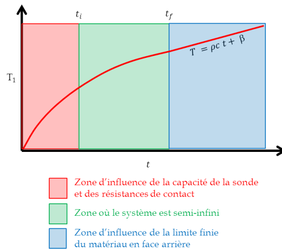
Figure II.11 : Illustration de la zone linéaire de la température du plan chaud isolé.
