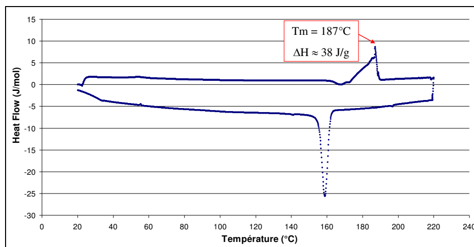
Figure V.II : Thermogramme de DSC du polyamide 11 diCOOH 5000
