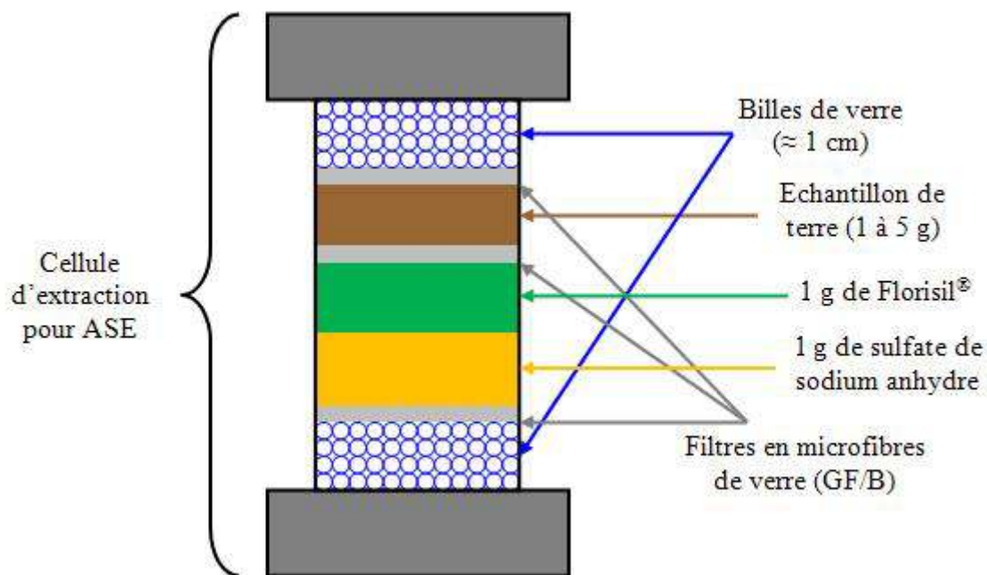
Figure II-14 : Schéma d'une cellule d'extraction préparée
