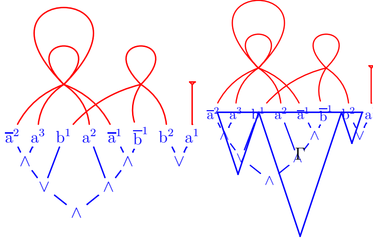
FIGURE 4 – Représentation graphique d'un F-préréseau (à gauche) et la représentation générique "glaçon/stalactite" d'une forêt de séquents (à droite)
