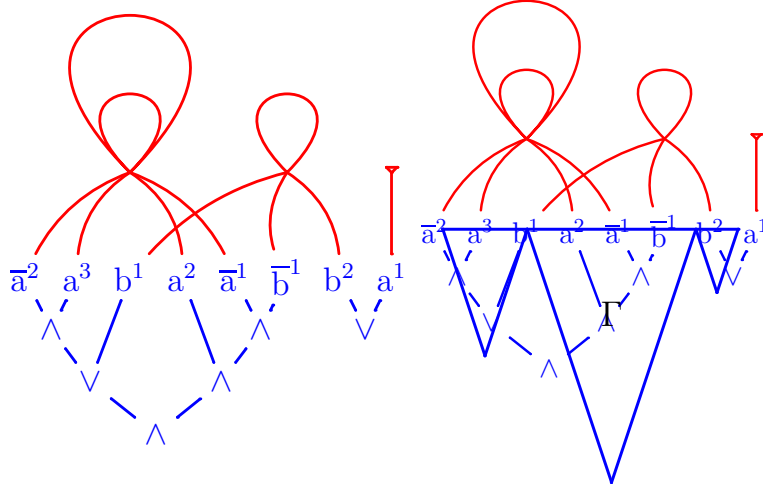
FIGURE 4 – Représentation graphique d'un F-préseau (à gauche) et la représentation générique "glaçon/stalactite" d'une forêt de séquents (à droite)
