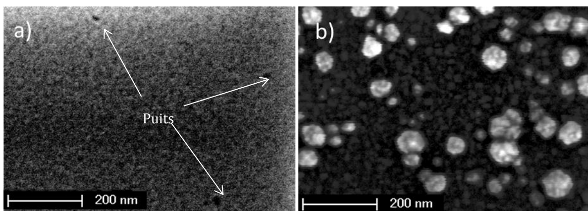
Figure III-11 : Micrographies MEB à 1 mm des bords d'échantillons ayant subi une étape de polarisation à 2 % de méthane d'une durée de 30 s pour la première a) et de 6 min pour la seconde b).
