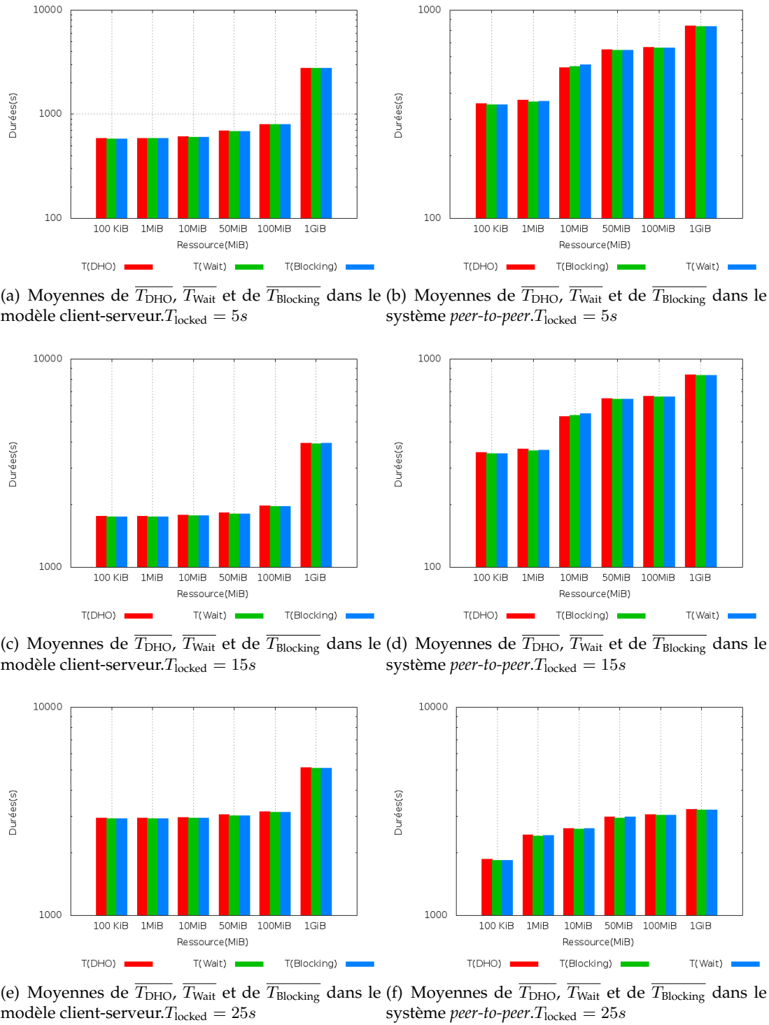
FIGURE 6.8 – Comparaison des durées moyennes \overline{T_{DHO}} , \overline{T_{Wait}} et \overline{T_{Blocking}} entre le modèle centralisé et le système peer-to-peer en diversifiant la taille de la ressource et le temps applicatif T_{locked}
