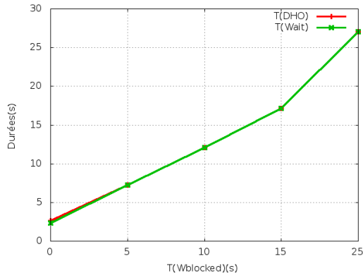
(a) Durées moyennes en fonction du délai T_{\text{Wblocked}} pour une occupation de 0(s) en section critique
