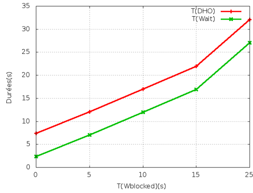
(b) Durées moyennes en fonction du délai T_{\text{Wblocked}} pour une occupation de 5(s) en section critique
