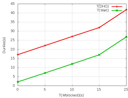
(c) Durées moyennes en fonction du délai T_{\text{Wblocked}} pour une occupation de 15(s) en section critique
