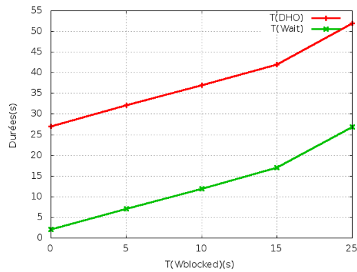
(d) Durées moyennes en fonction du délai T_{\text{Wblocked}} pour une occupation de 25(s) en section critique
